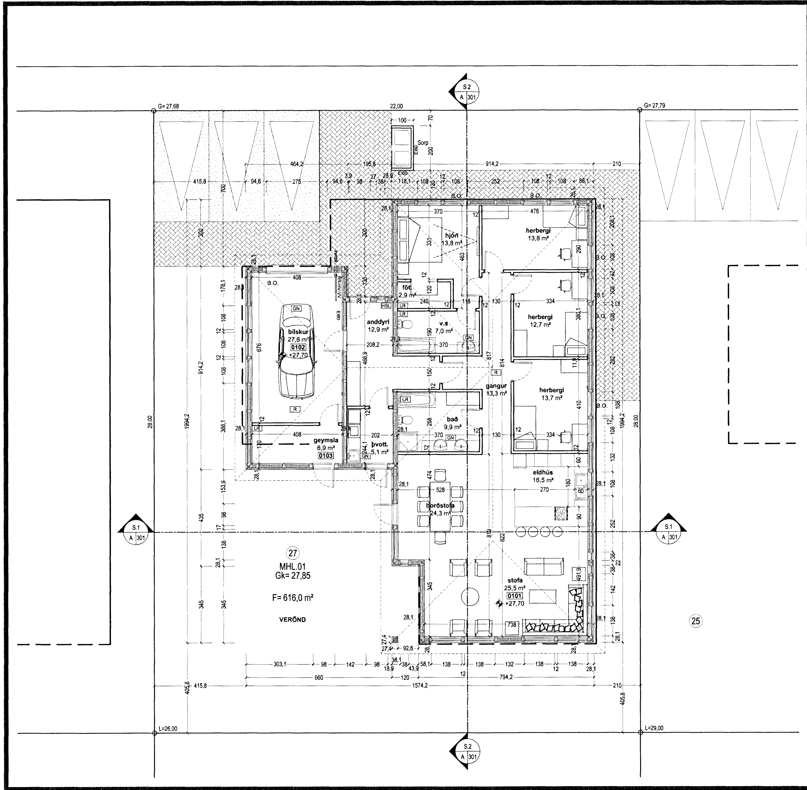
Grunmynd 1:100
