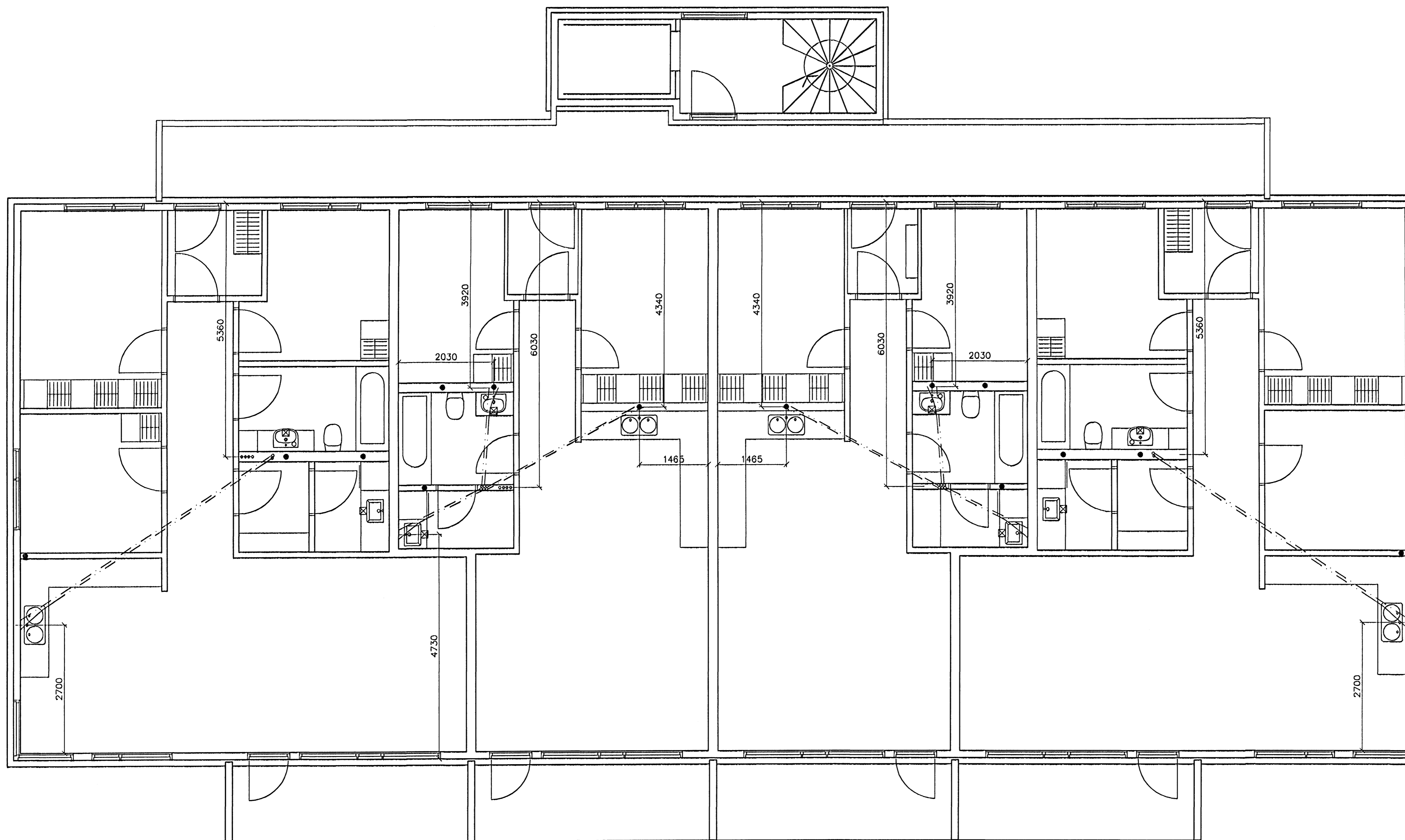
GRUNNMYND 2 HÆÐAR 1:50
