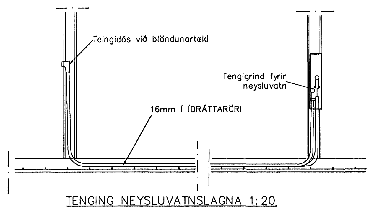
TENGING NEYSLUVATNSLAGNA 1:20
