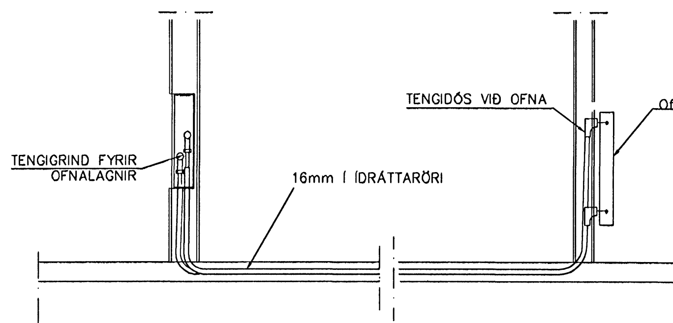
TENGING OFNALAGNALAGNA 1:20
