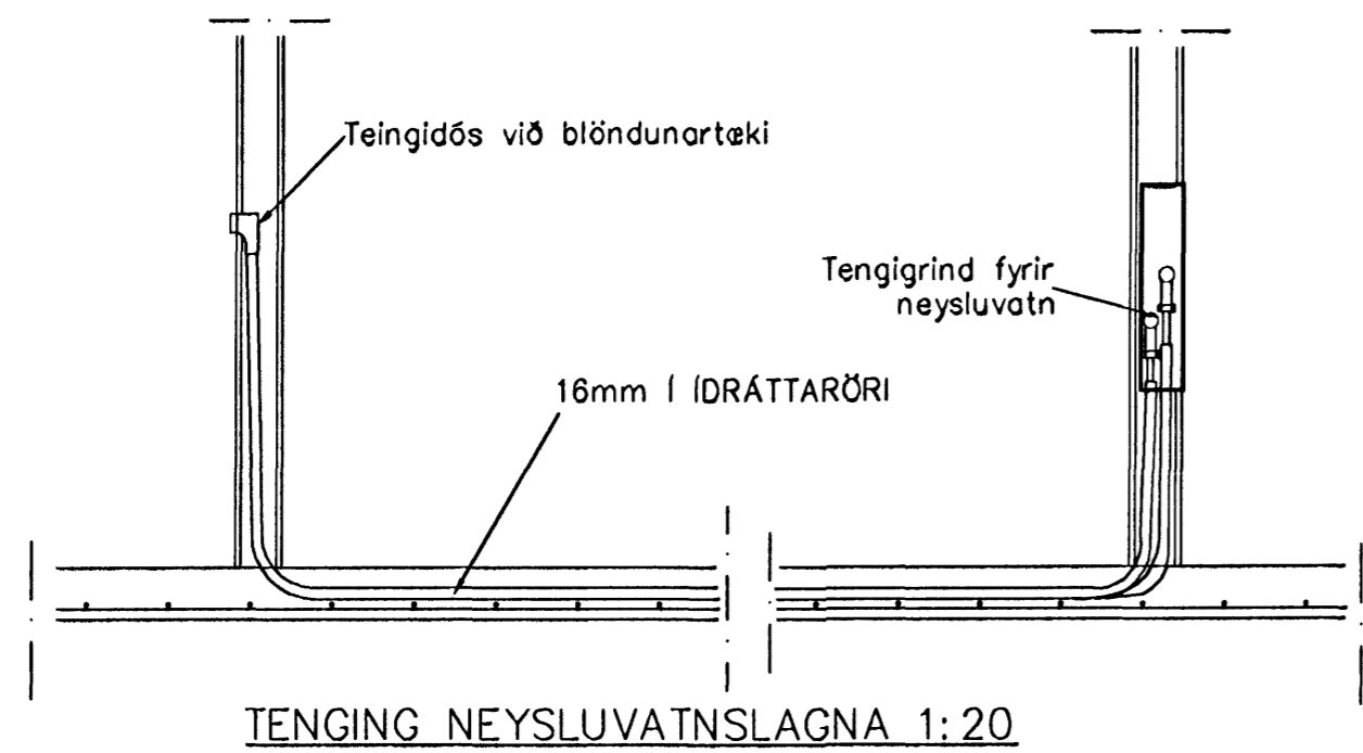
TENGING NEYSLUVATNSLAGNA 1:20
