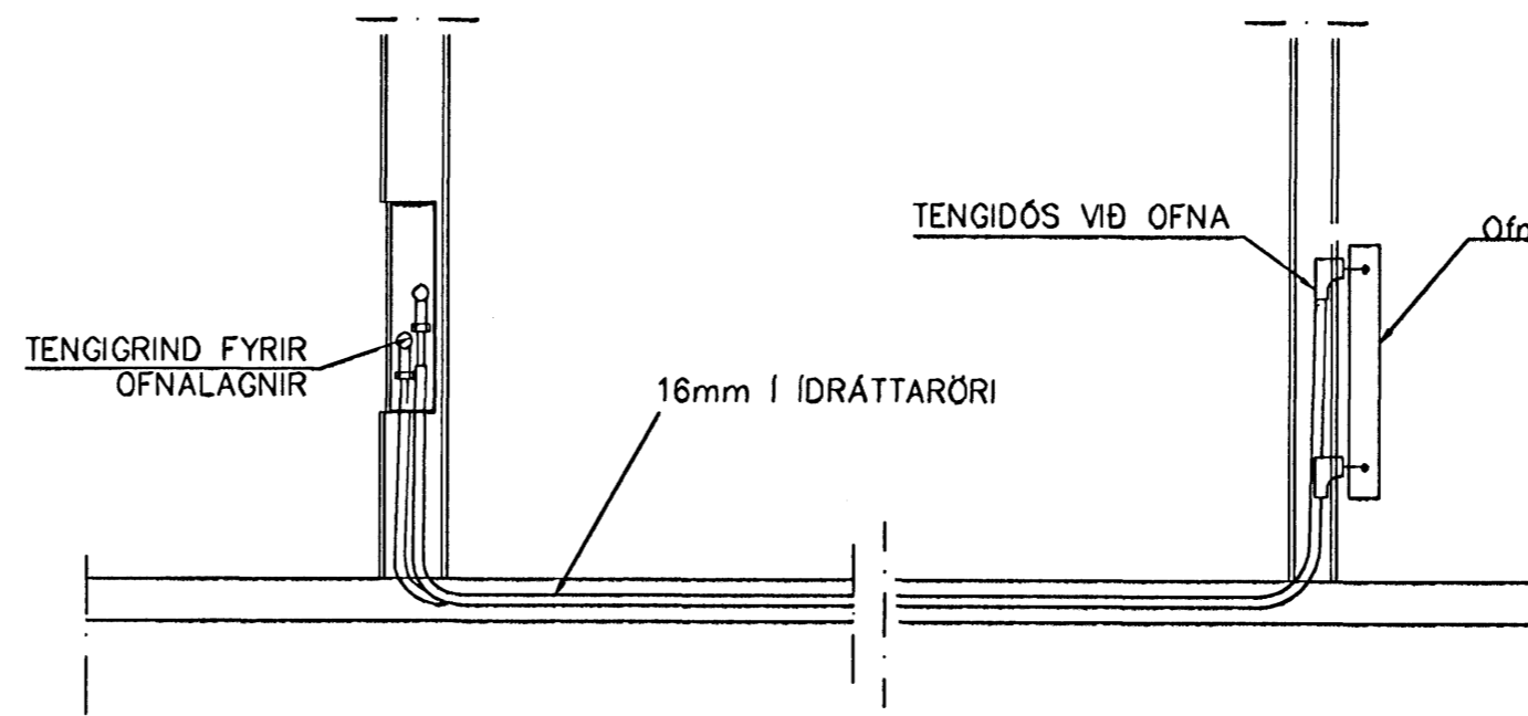
TENGING OFNALAGNALAGNA 1:20
