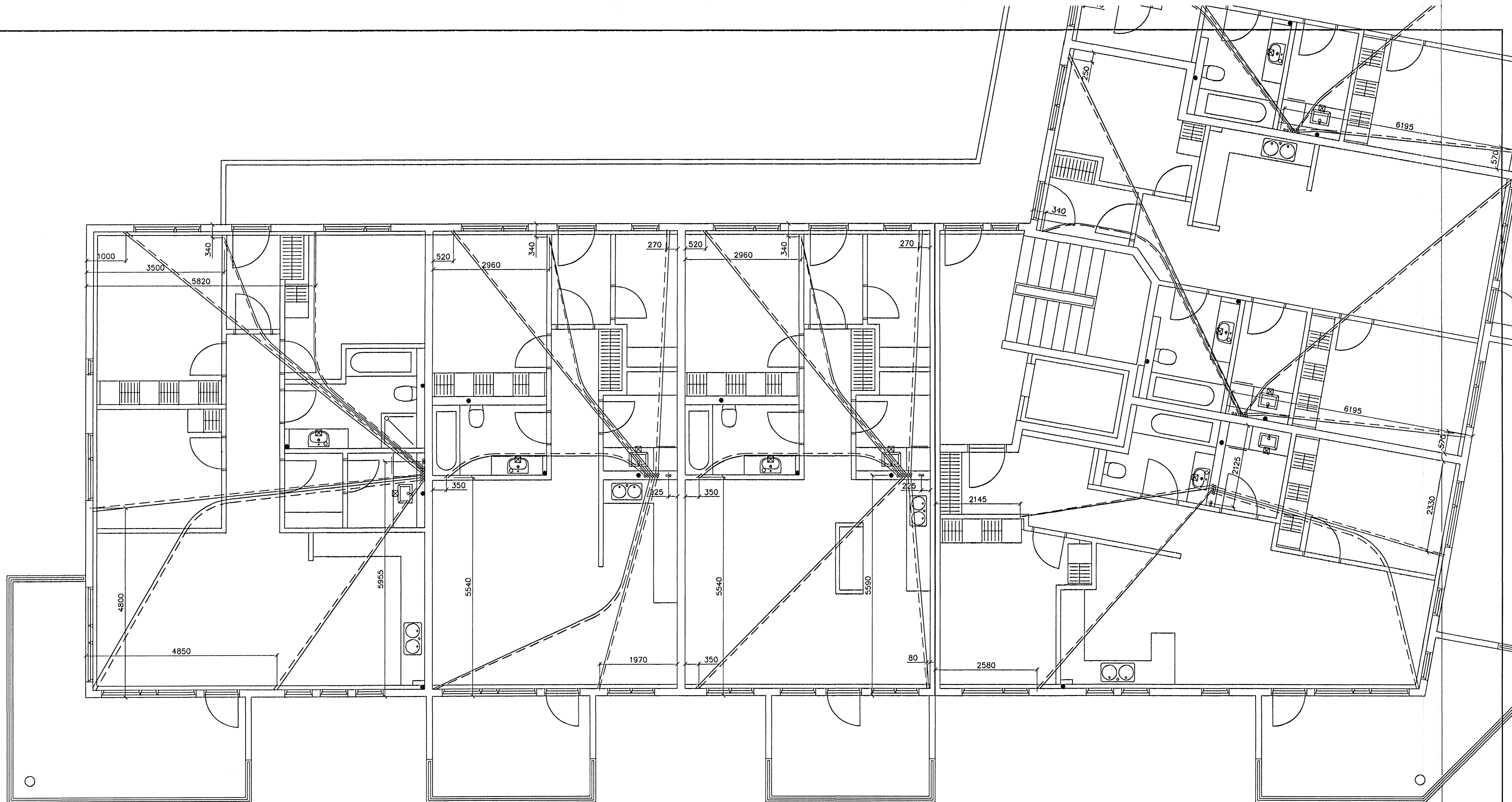
GRUNNMYND 5 HÆÐAR 1:50
