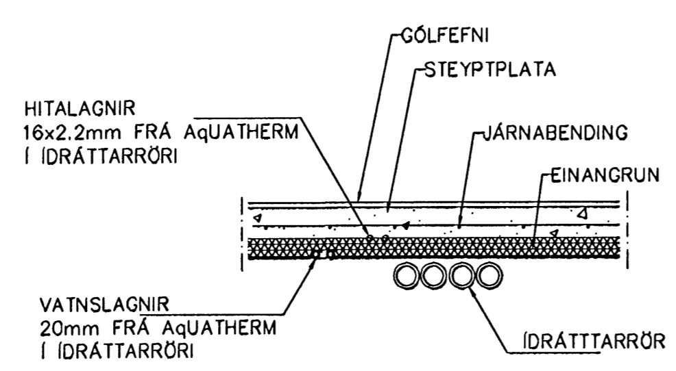
LAGNIR, SNIÐ, 1:20
