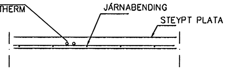
LAGNIR, SNIÐ, 1:20
