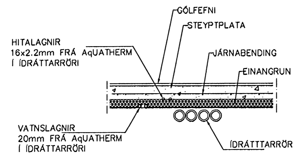
LAGNIR, SNIÐ, 1:20
