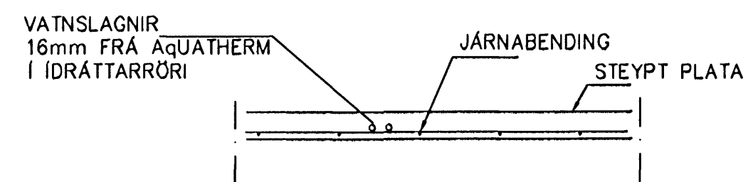
LAGNIR, SNIÐ, 1:20
