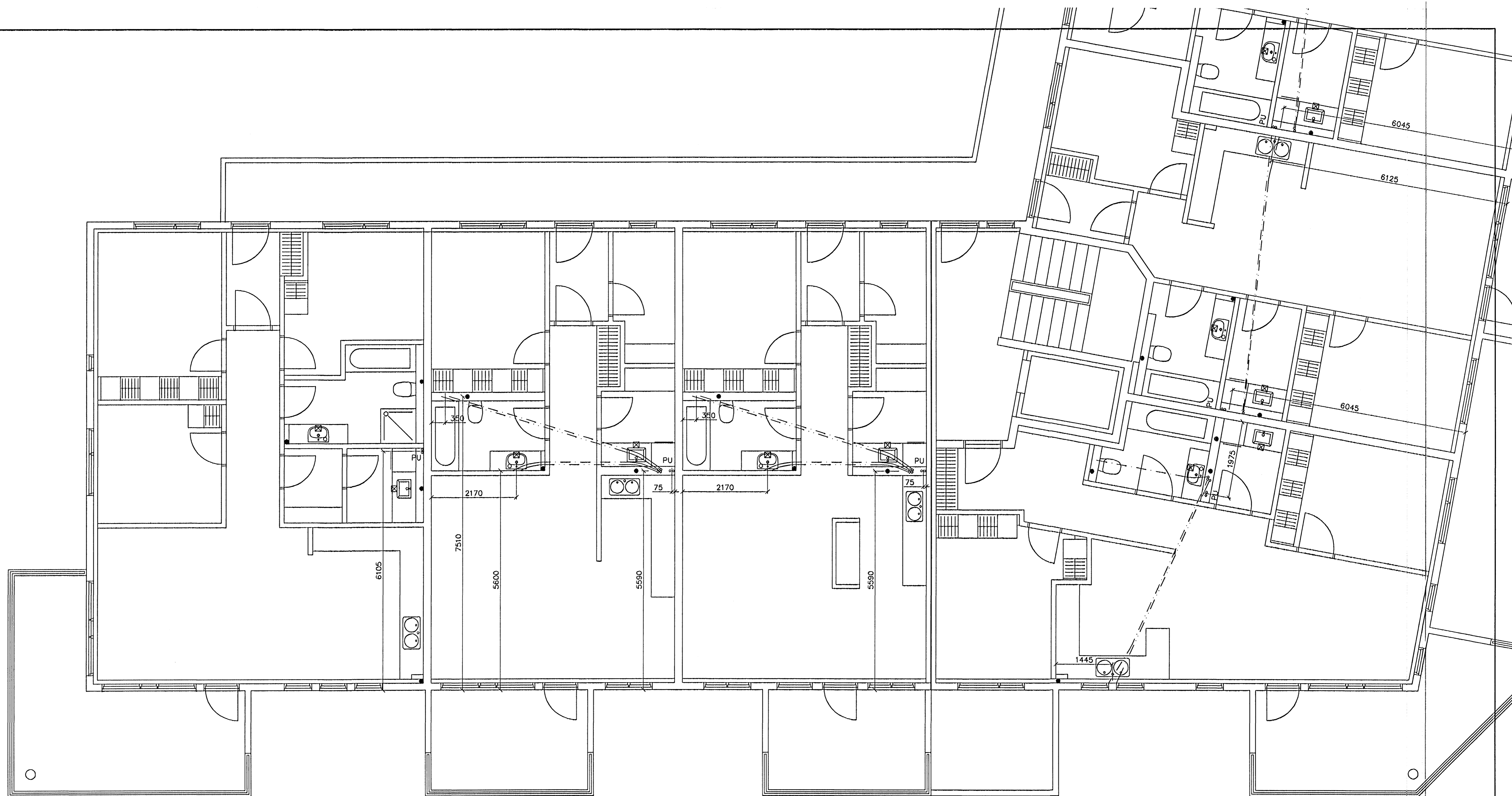
GRUNNMYND 2 HÆÐAR 1:50
