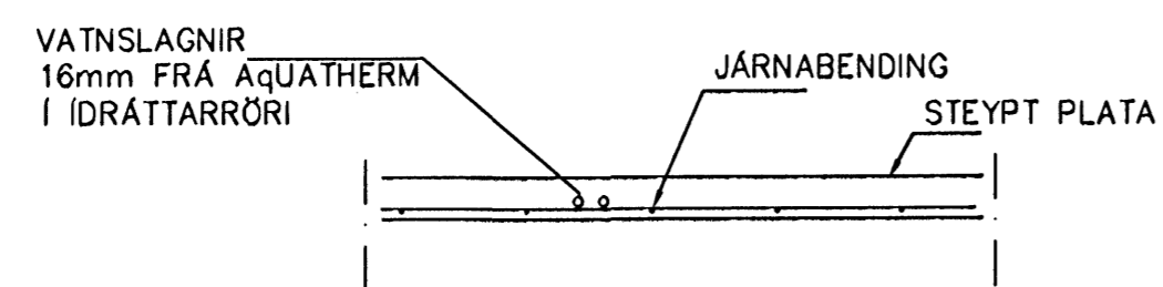
LAGNIR, SNIÐ, 1:20
