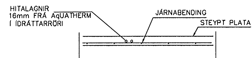
LAGNIR, SNIÐ, 1:20
