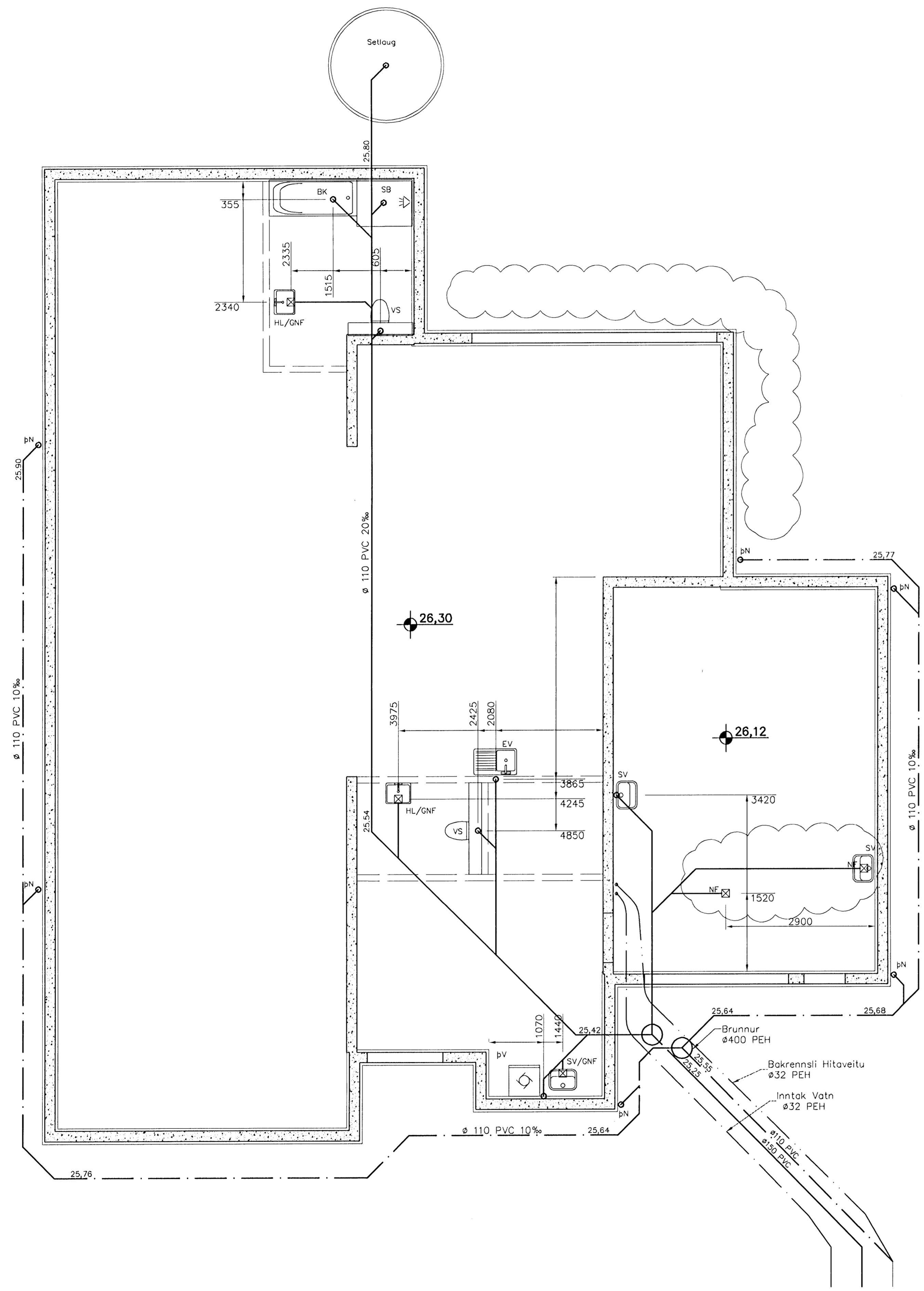
Grunnlagir 1:50
