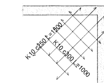
A MERKIR JÄRNBENDINGU Í HORNUM
