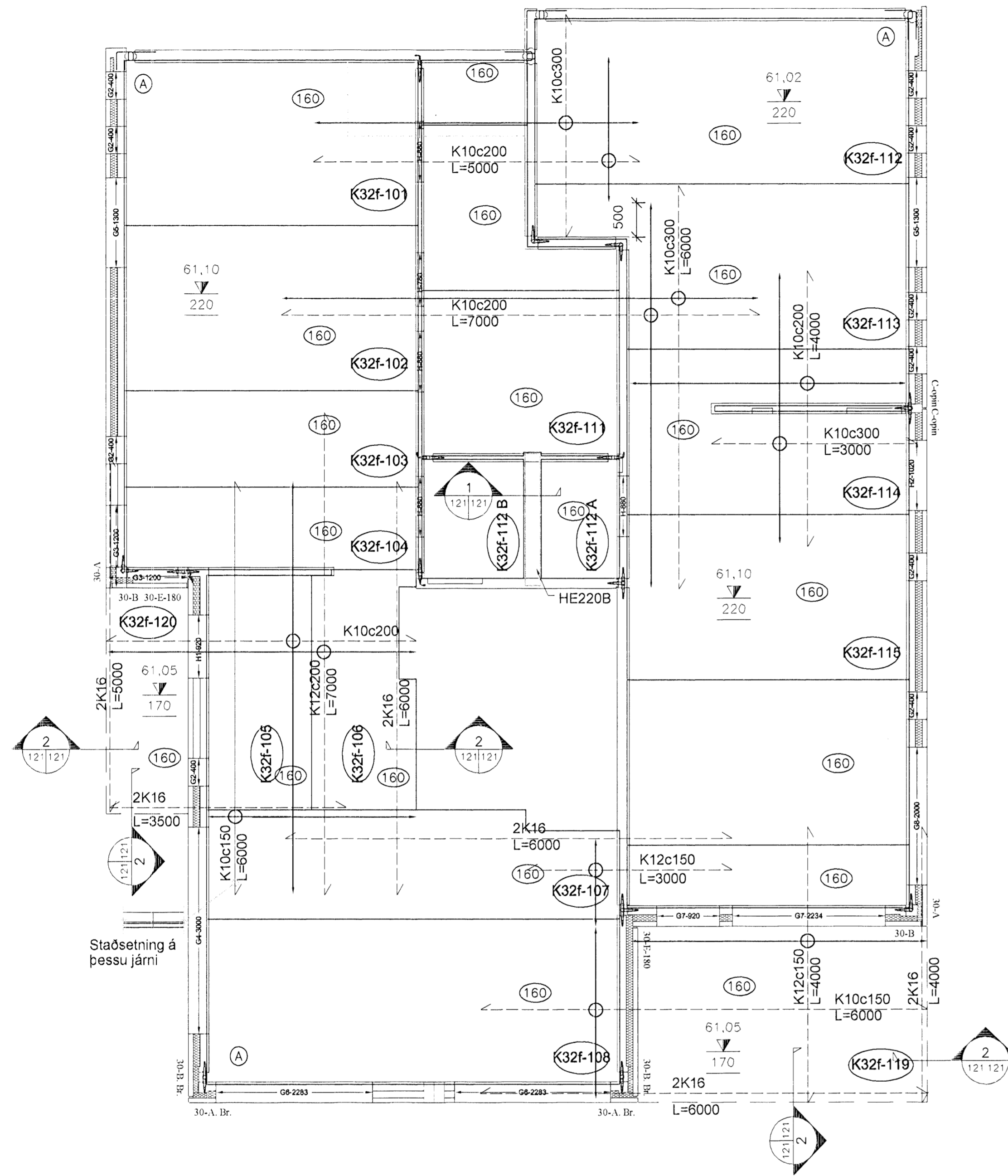
GRUNNMYND - LOFTAPLÖTUR, EFRI JÄRNBENDING PLATA YFIR 1 HÆÐ 1:50
