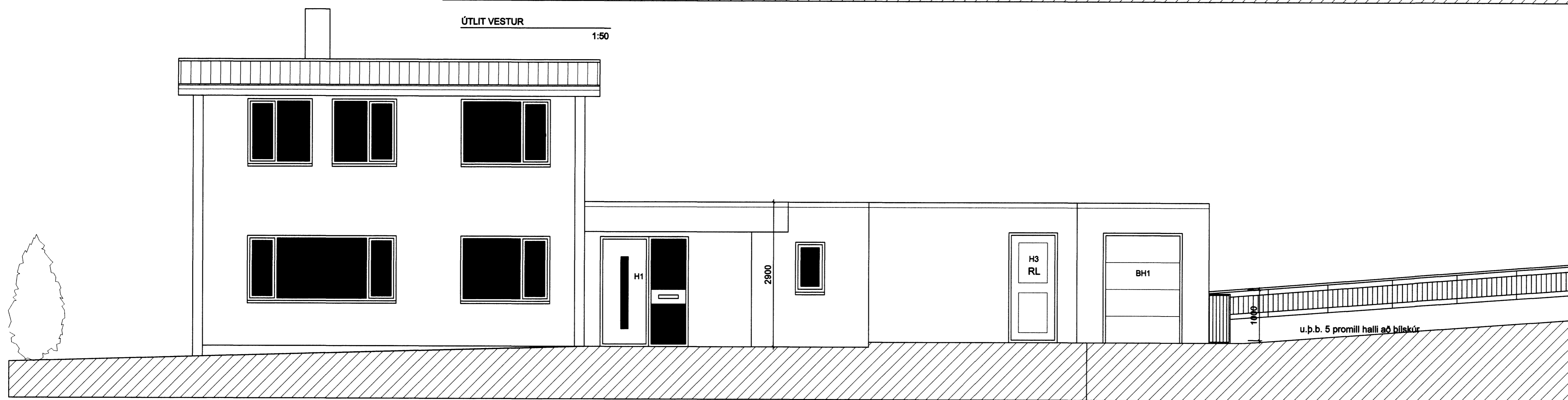
ÚTLIT SUÐUR 1:50
