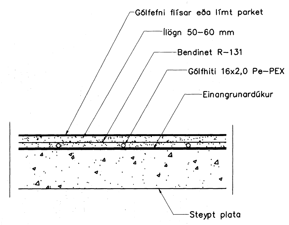
Gólfhiti snið, 1:10
