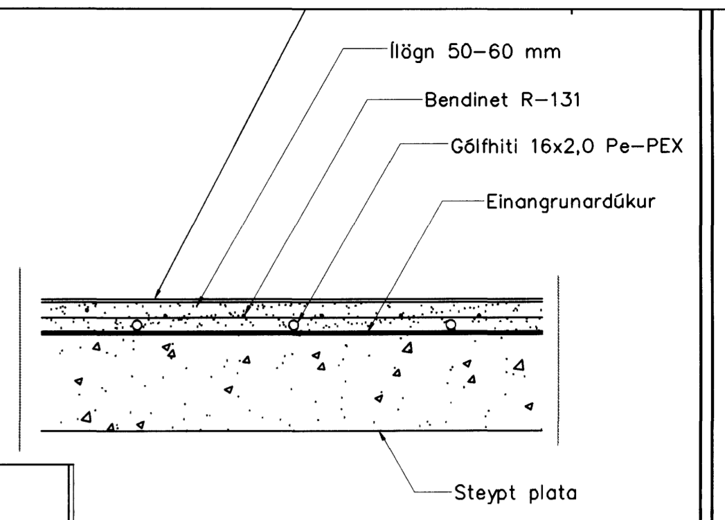
Gólfhiti snið, 1:10
