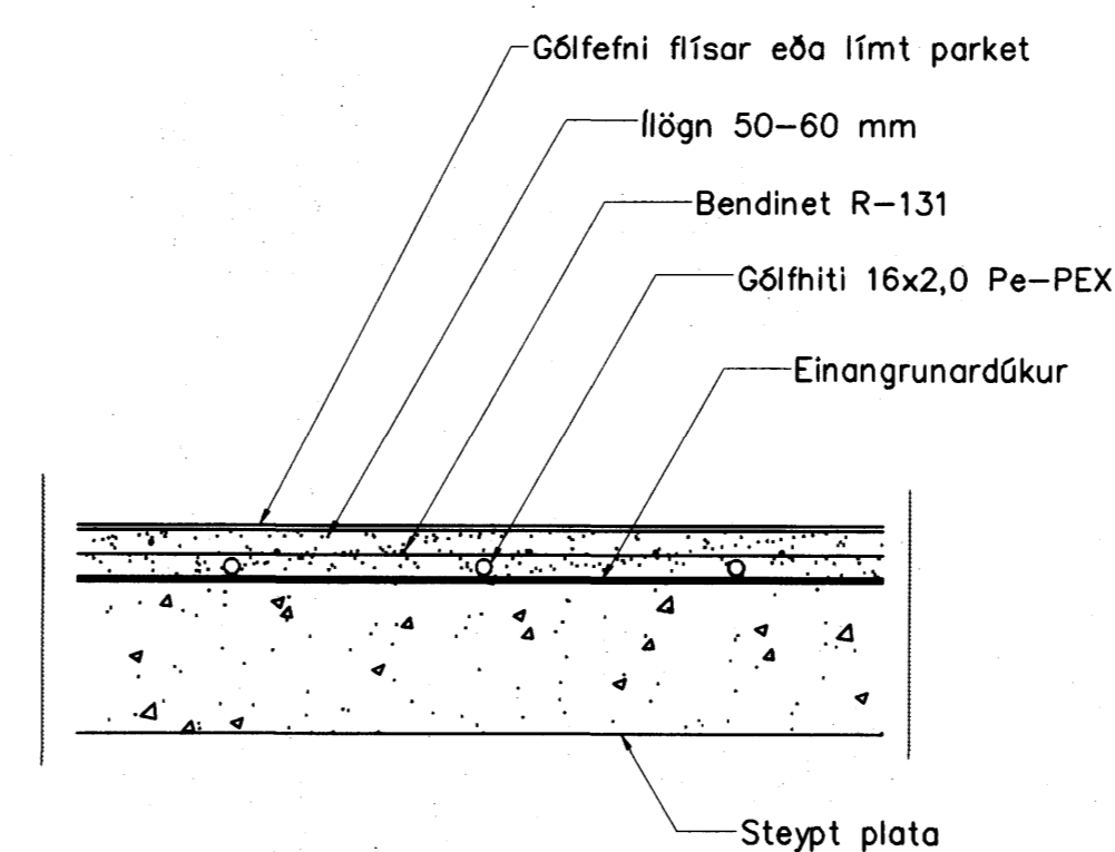
Gólfhiti snið, 1:10
