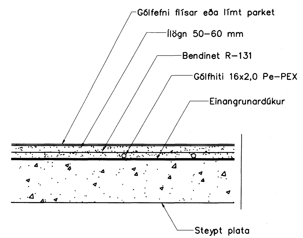
Gólfhiti snið, 1:10
