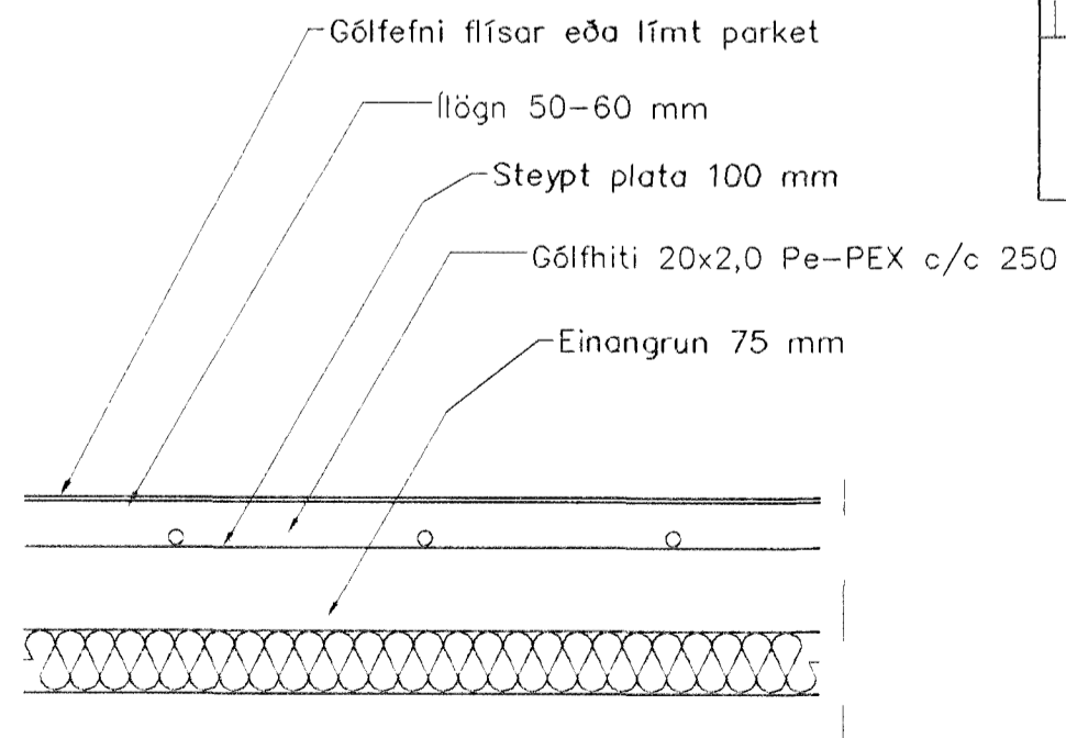
GÓLFHITI SNIÐ, 1:20
