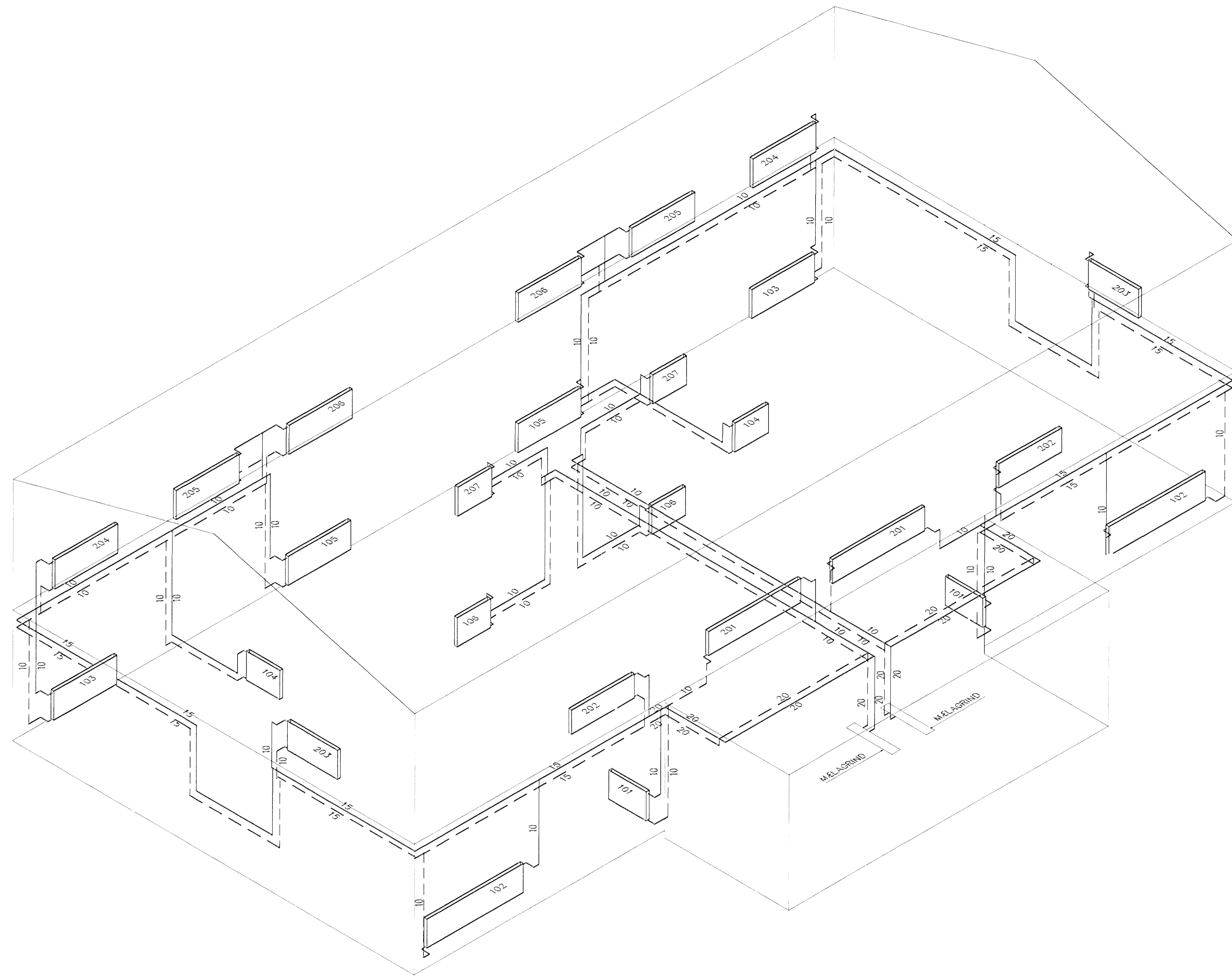
RÜMMYND HITLAGNA 1:50
