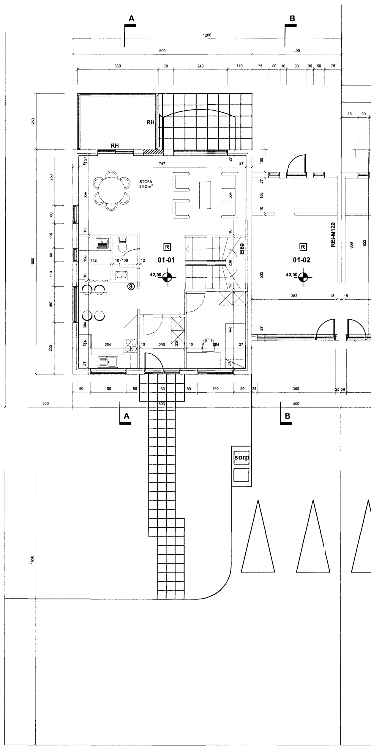
G=42.84 Grunnmynd 1.hæð mkv. 1:100 G=41.04
