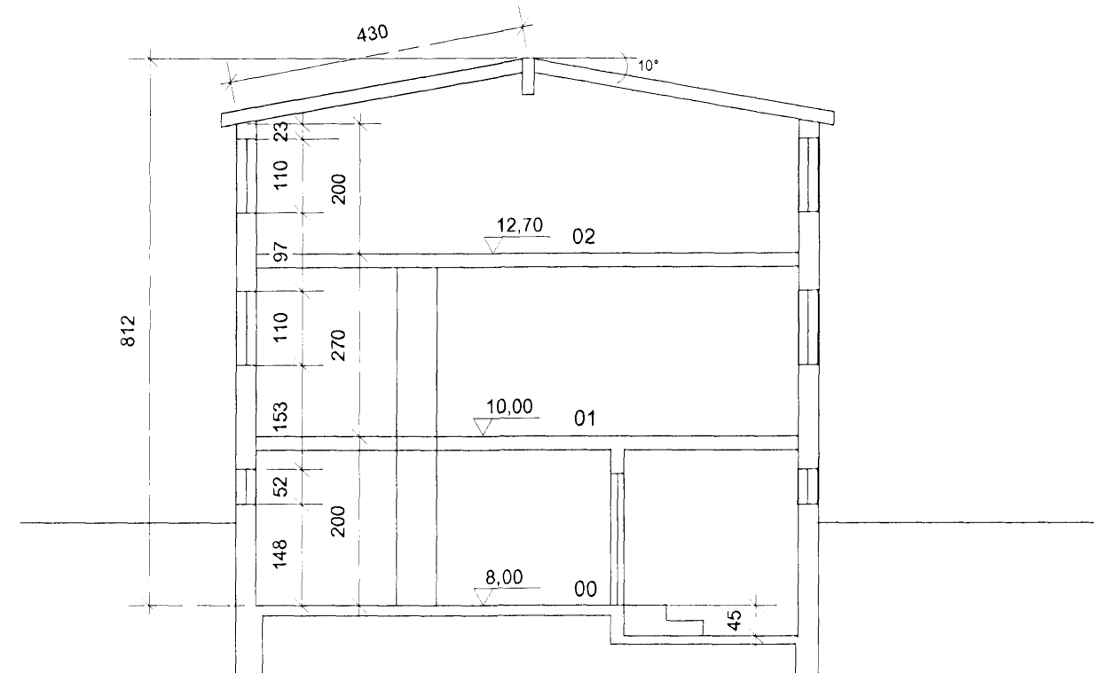
Snið A-A Mkv 1:100
