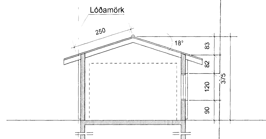
Snið B-B Mkv 1:100
