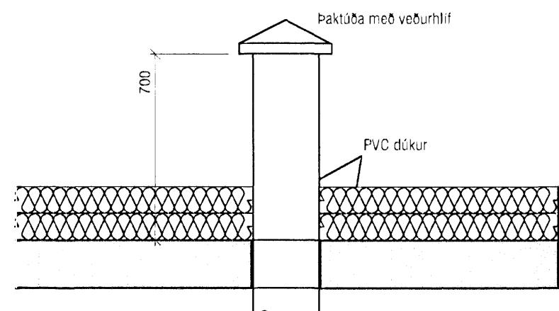
Snið í lofttúbu fyrir lyftu- og stígaúss 1:20
