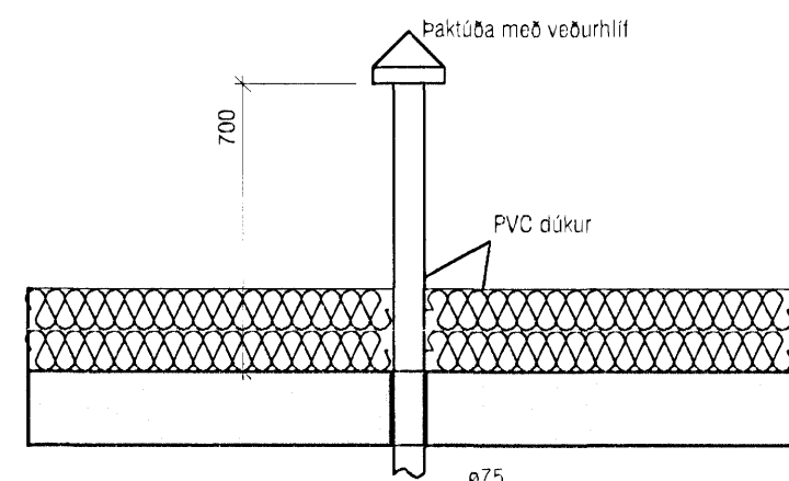
Snið í lofttúkur fyrir fallþípur 1:20
