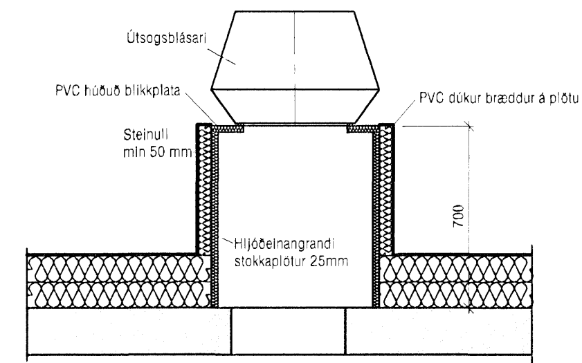
Snið í safnkassa og stokk á þaki
