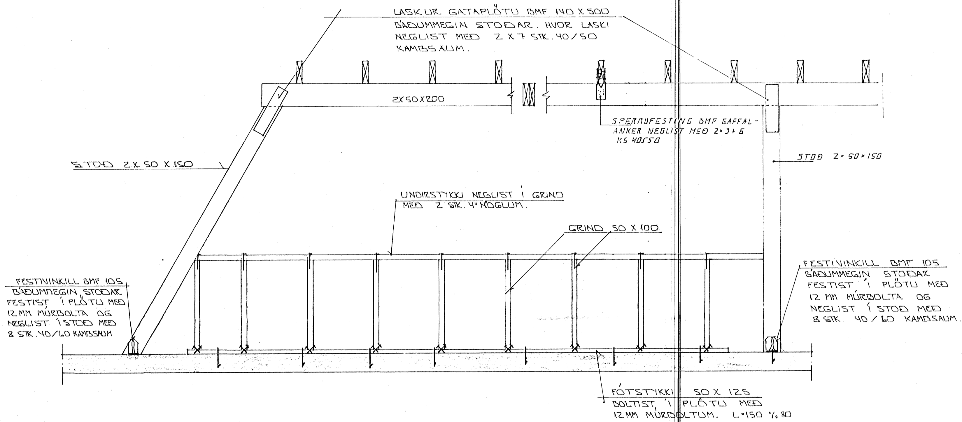
ASÝND A - A * 1:20
