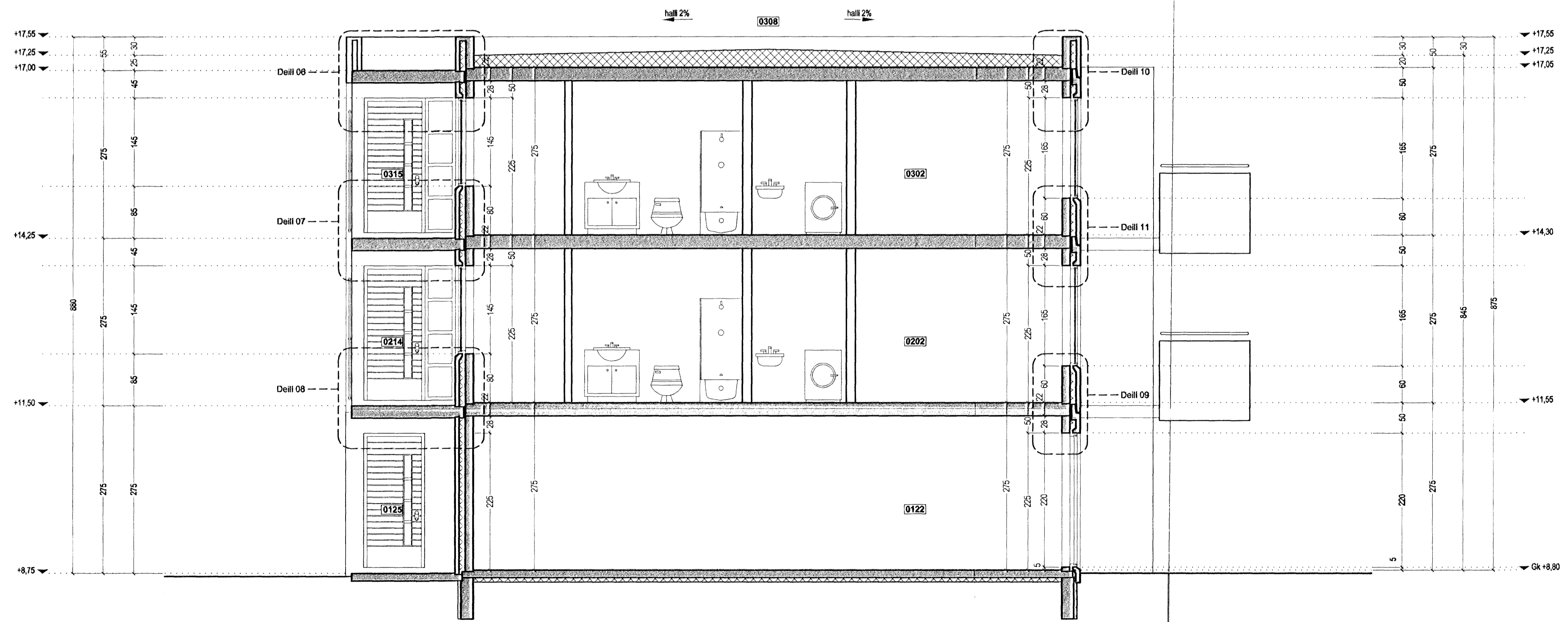
skurður C-C
