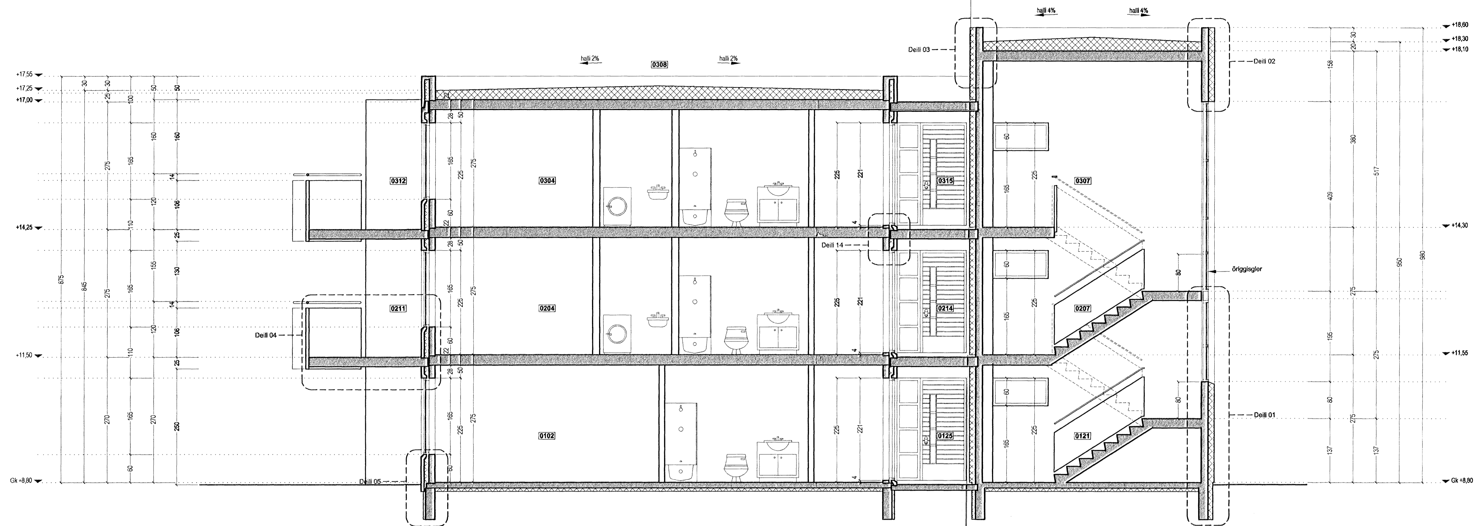
skurður B-B
