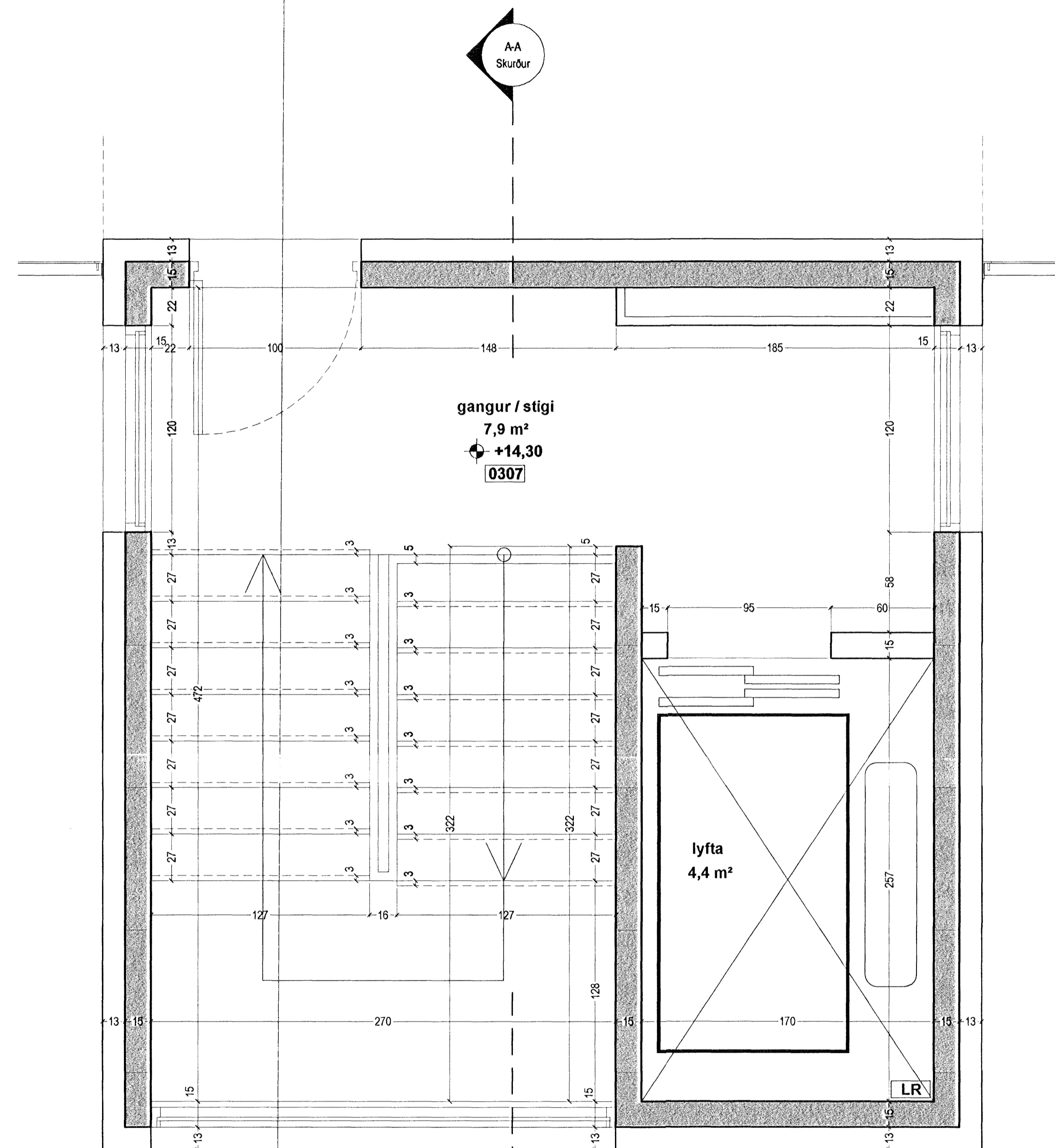
Grunnmynd 3.hæð
