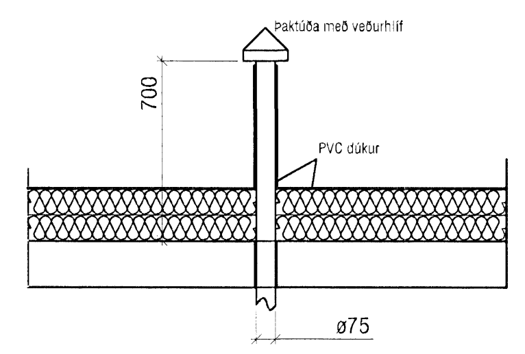
Snið í lofttúður fyrir fallþöpur. 1:20
