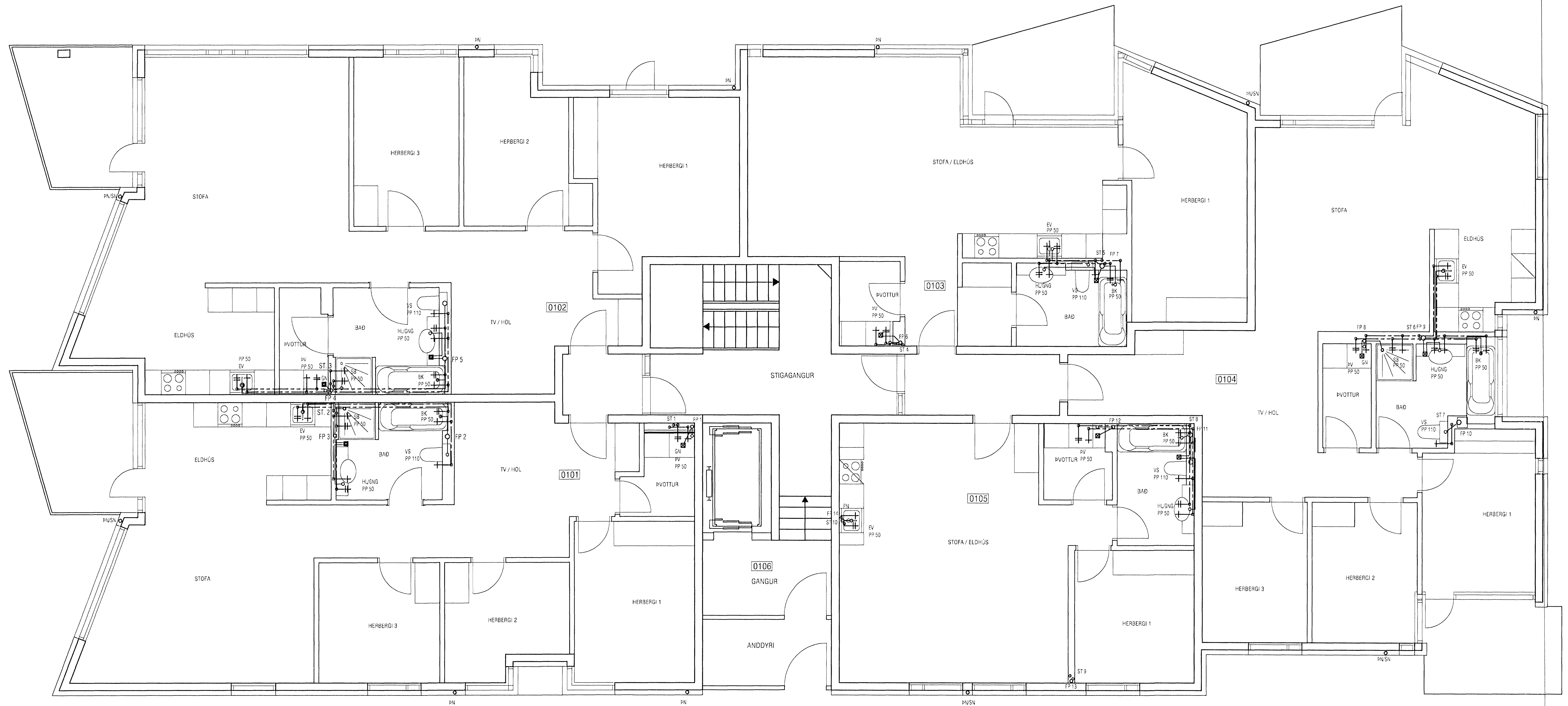
GRUNNMYND 1. HÆÐ
