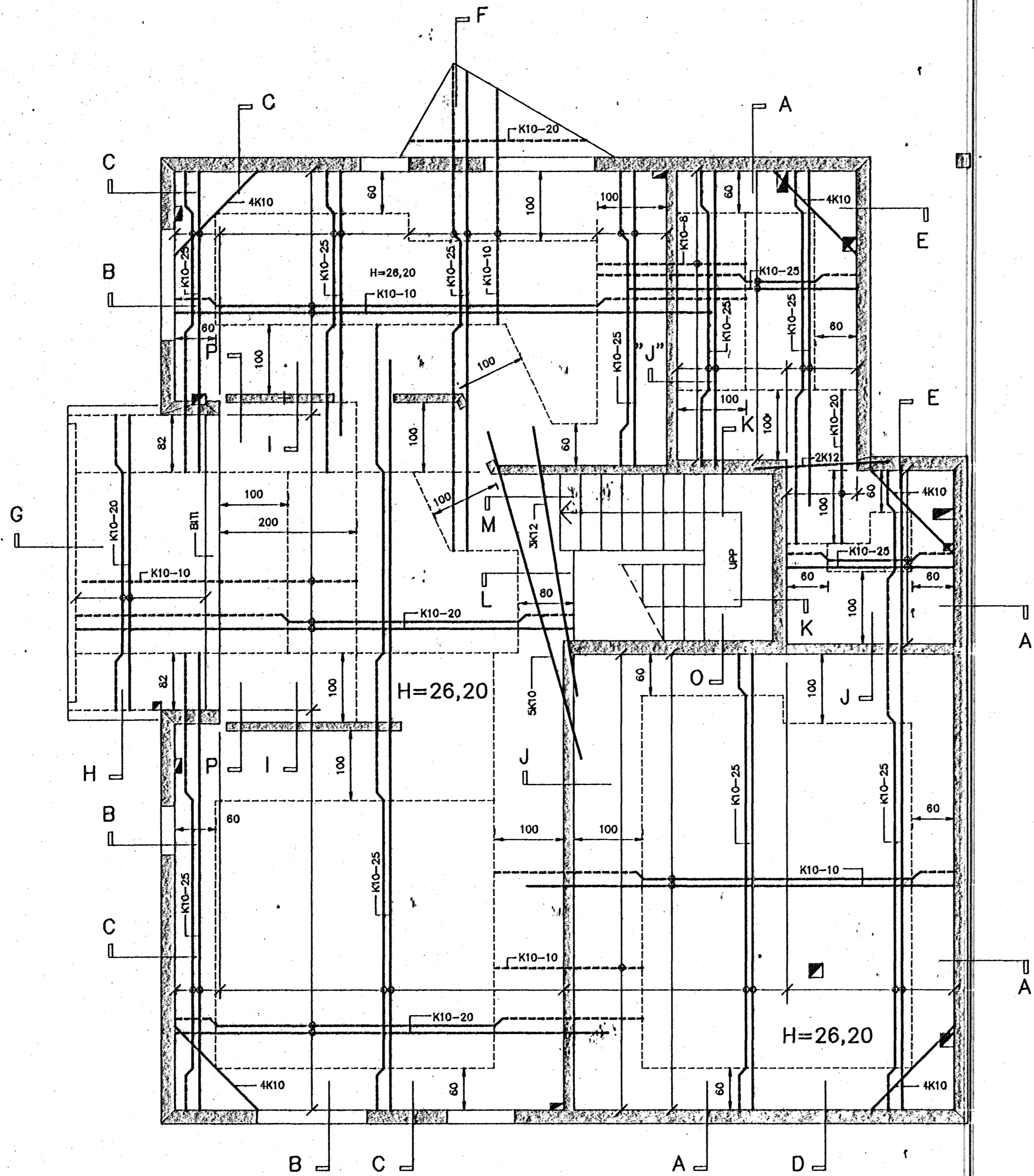
GRUNNMYND, M=1:50
