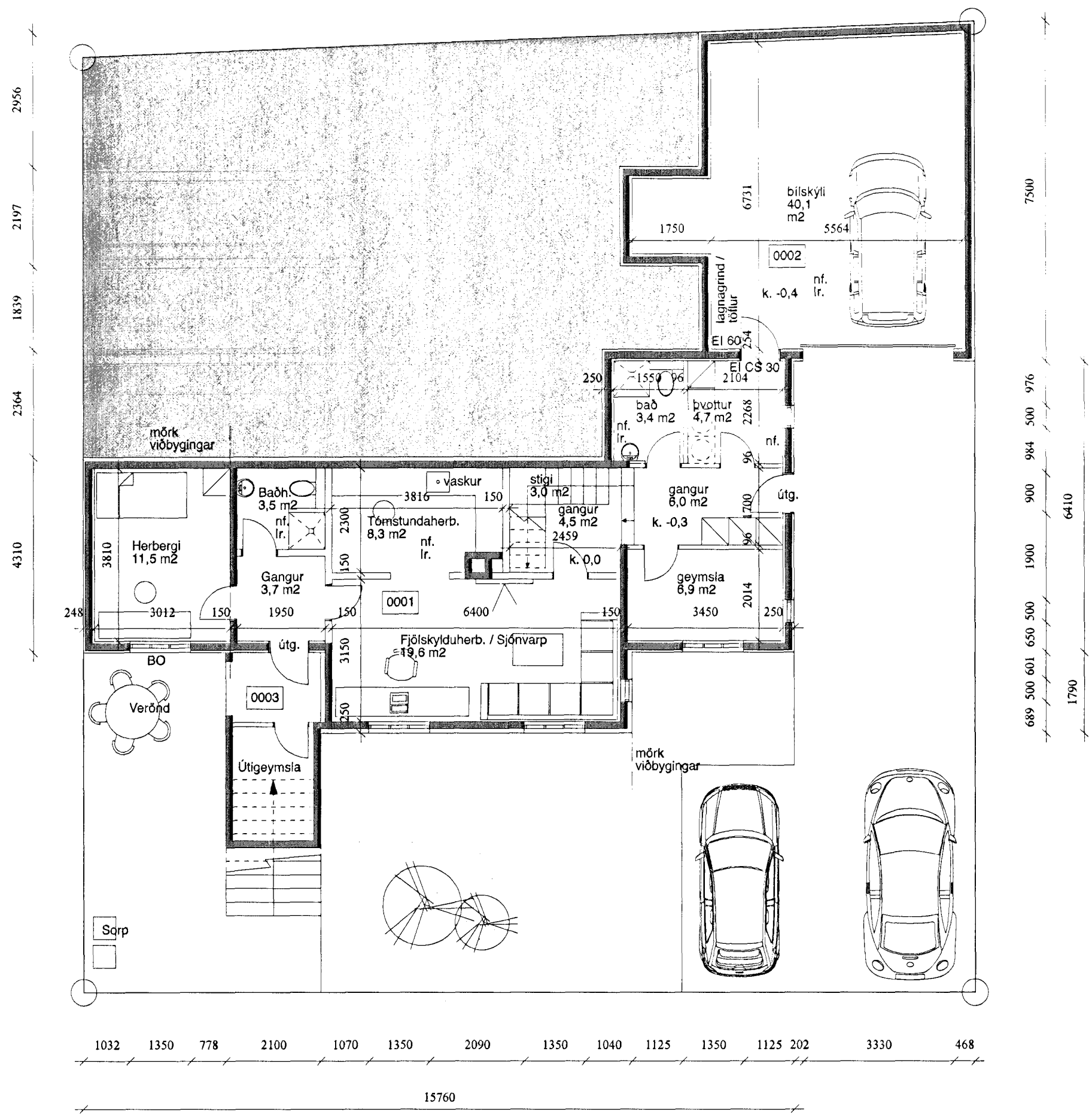
Grunnmynd neðri hæðar 1:100
