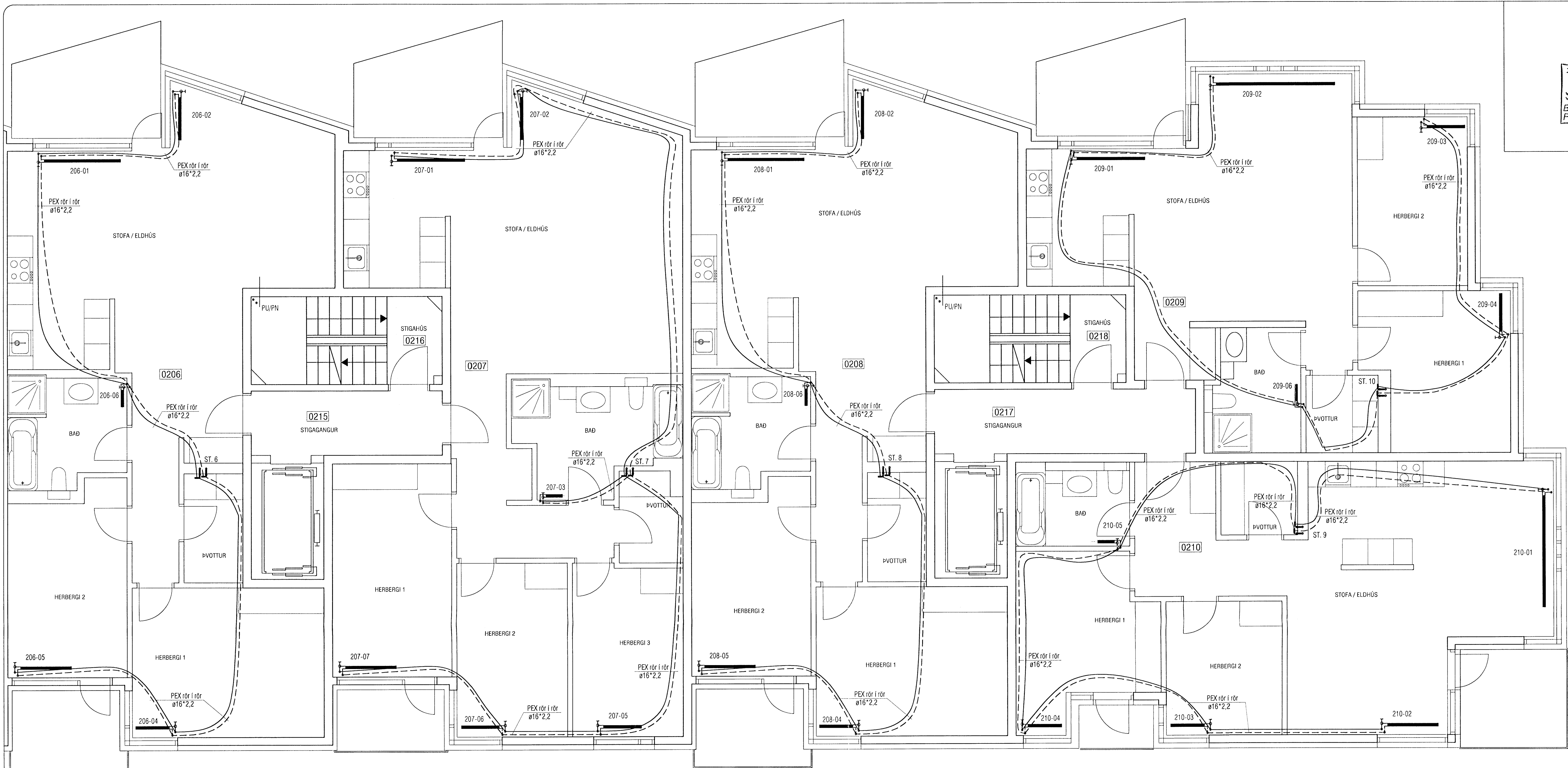
GRUNNMYND 2. HÆÐ NA
