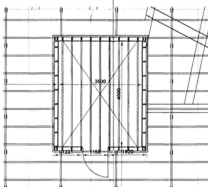
Tæknirými grunnmynd 1:100
