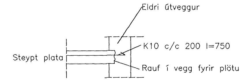
SNID A-A 1:20
