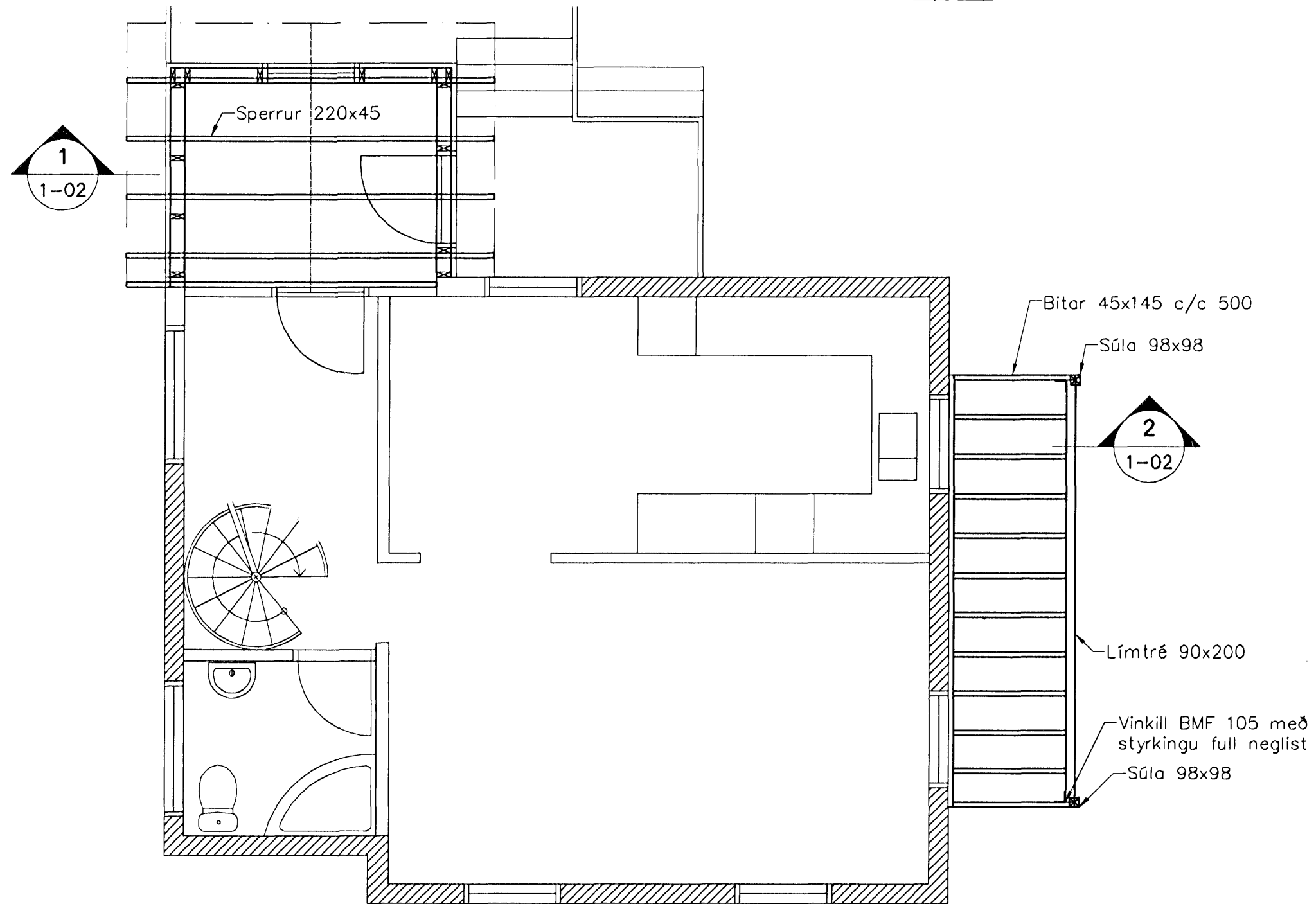
Grunnmynd, 1:50
