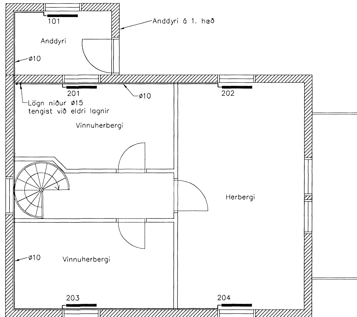
Rishæð, Grunnmynd, 1:50
