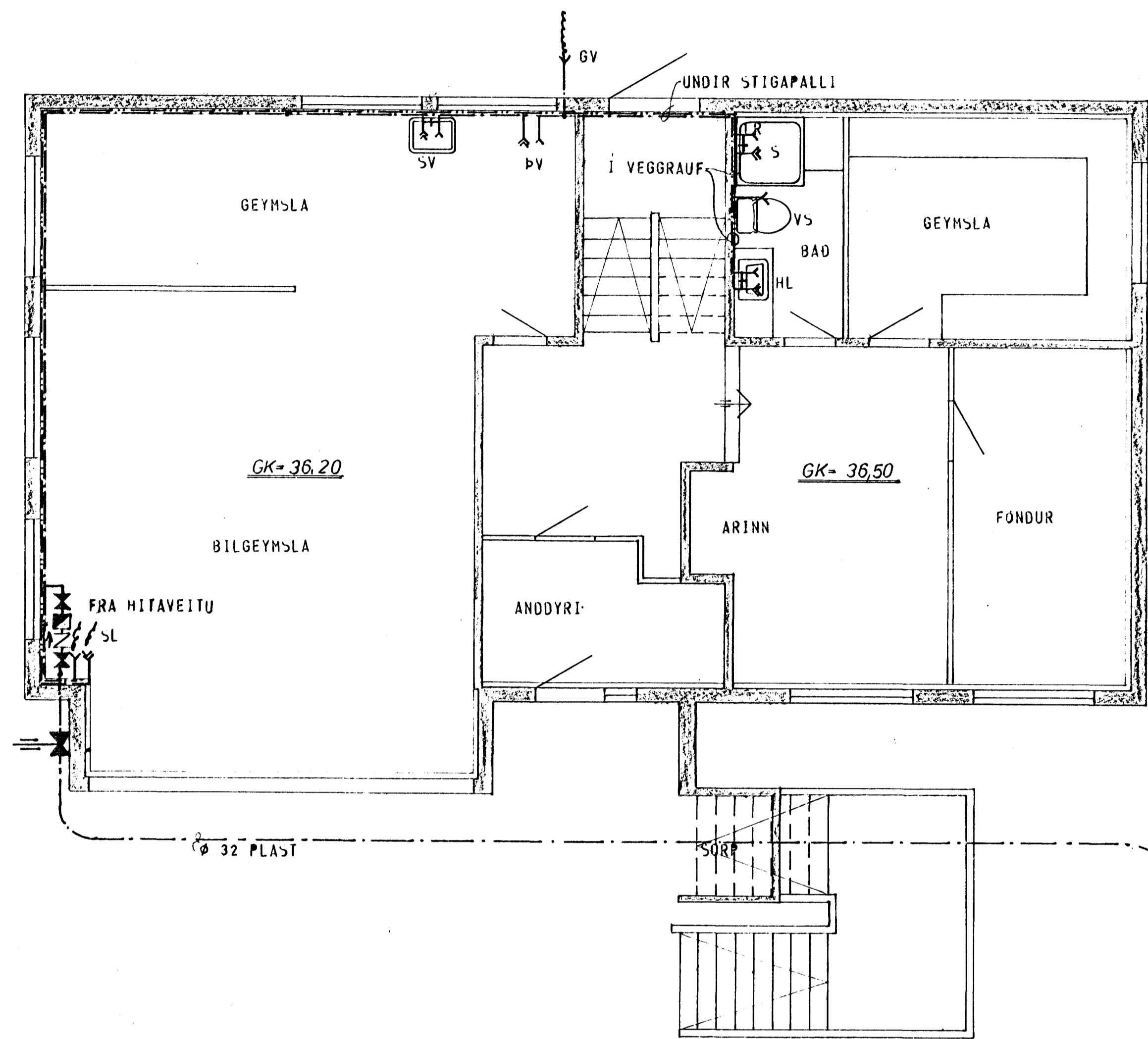
GRUNNMYND KJALLARA 1:50
