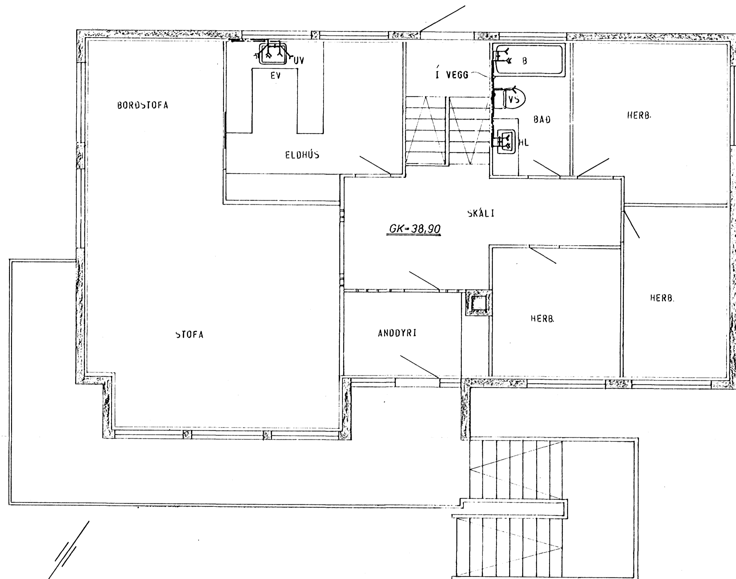
GRUNNMYND HÆÐAR 1:50
