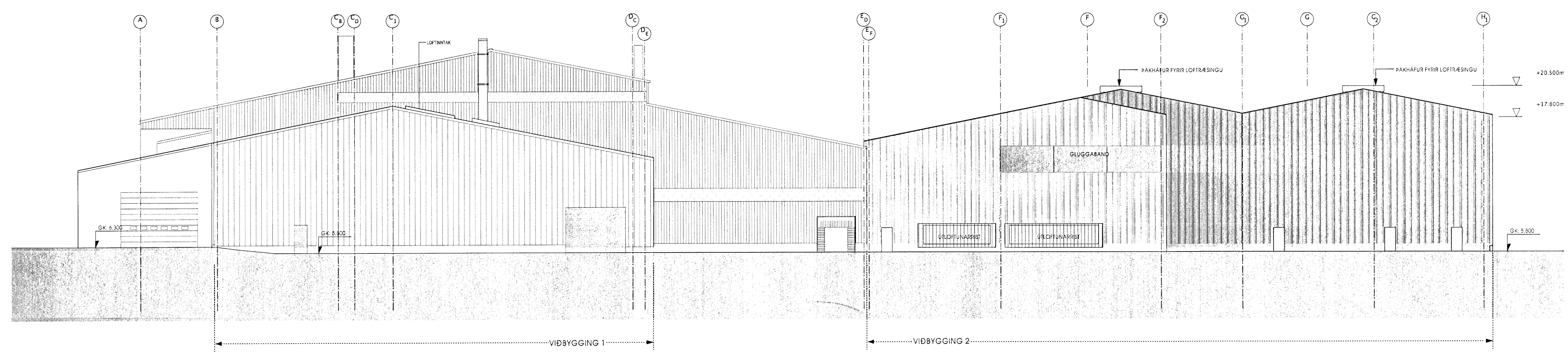
2 ÚTLIT AUSTUR / SNÍÐ Í GEGNUM BYGGINGU 1 m.kv. 1:200
