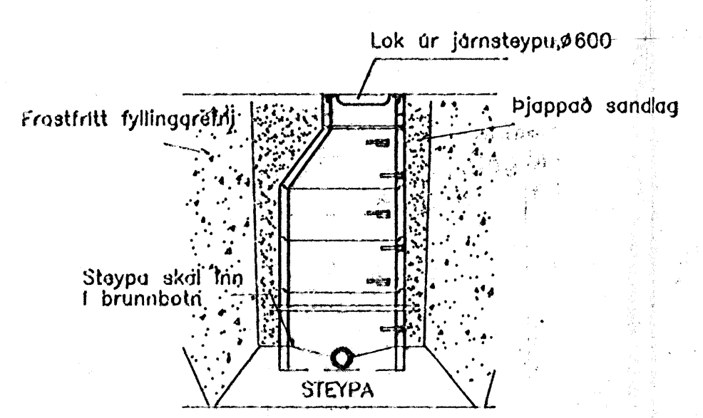
Þversnið í 1000 mm brunni M. 1:50
