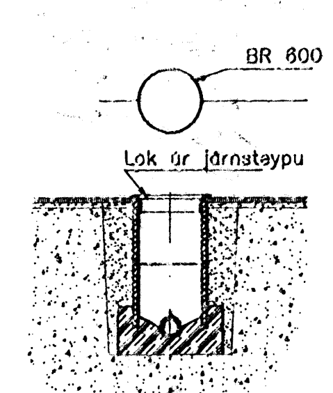
Frágangur \varnothing 600 brunns M. 1:50
