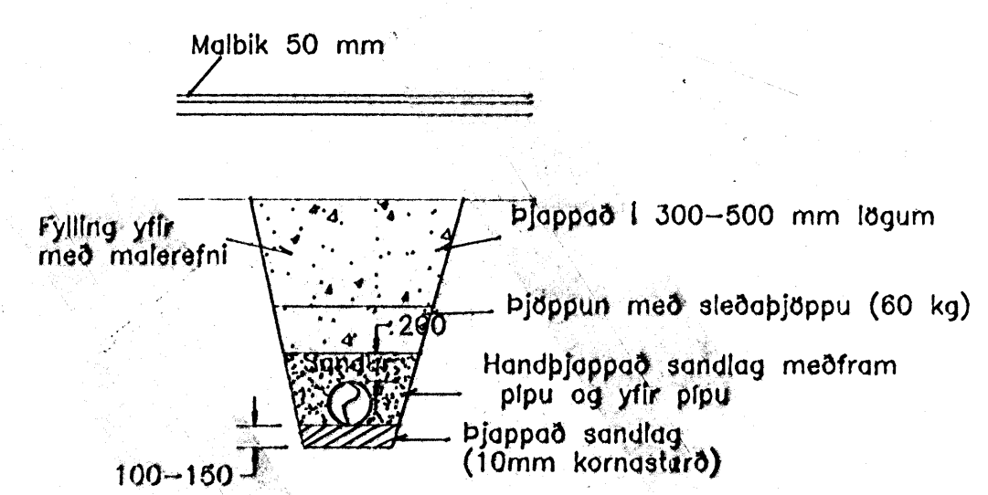
Þversnið í pípuskurð M. 1:50
