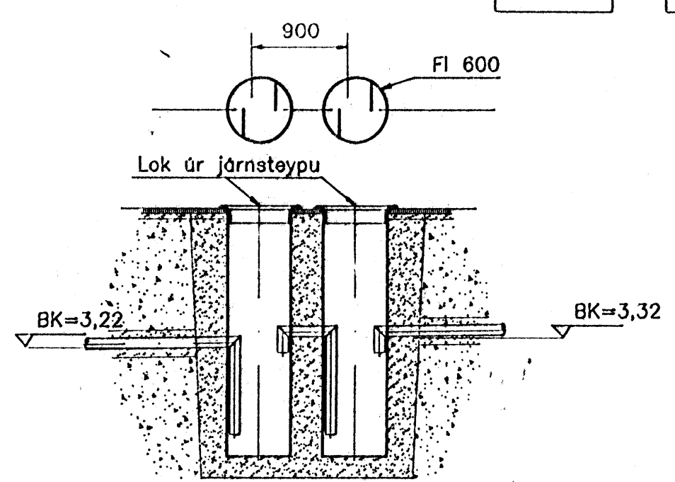
Þversnið í fitugildru M. 1:50
