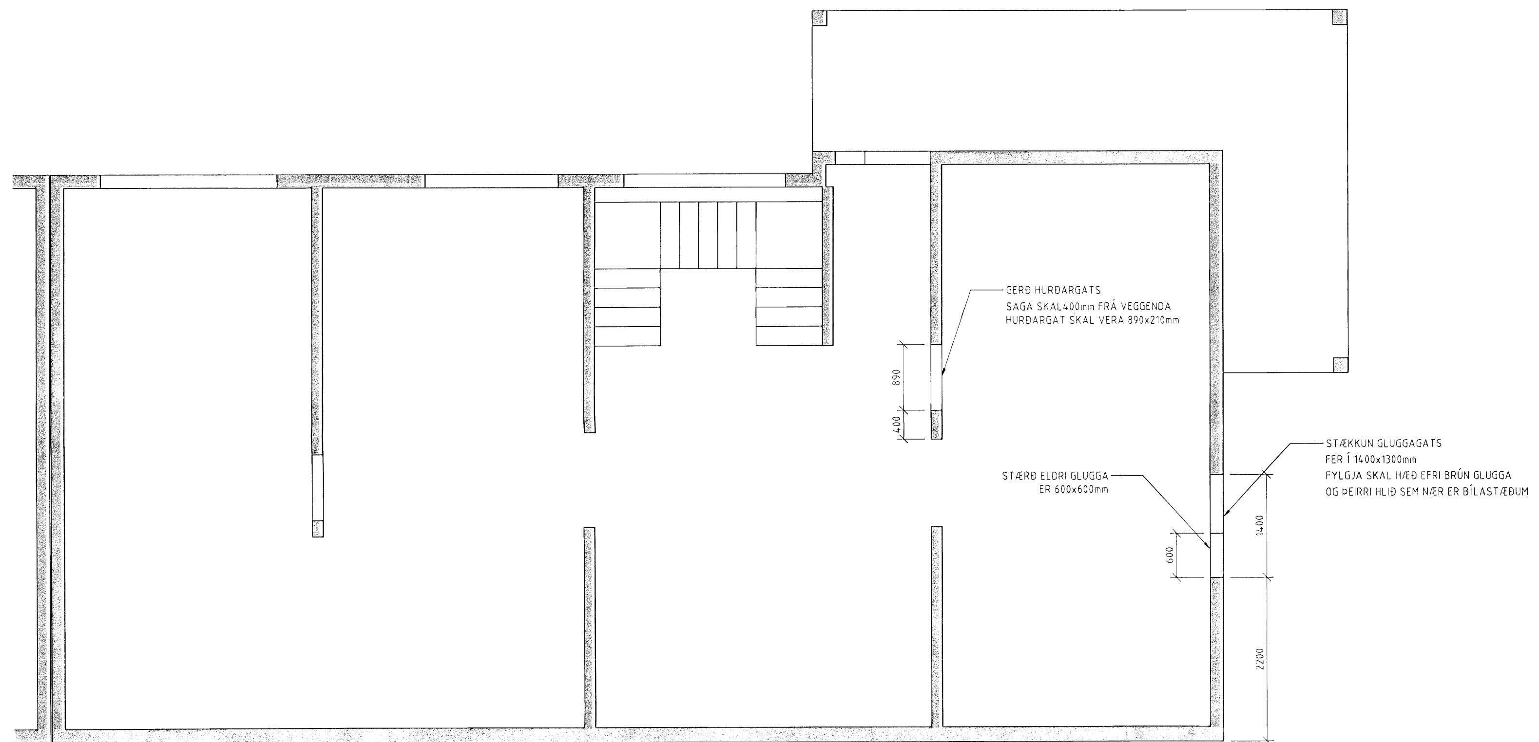
GRUNNMYND, NEDRI HÆÐAR 150 ÚRSÖGUN HURDARGATS OG GLUGGAGATS HLÍÐARÁS 5
