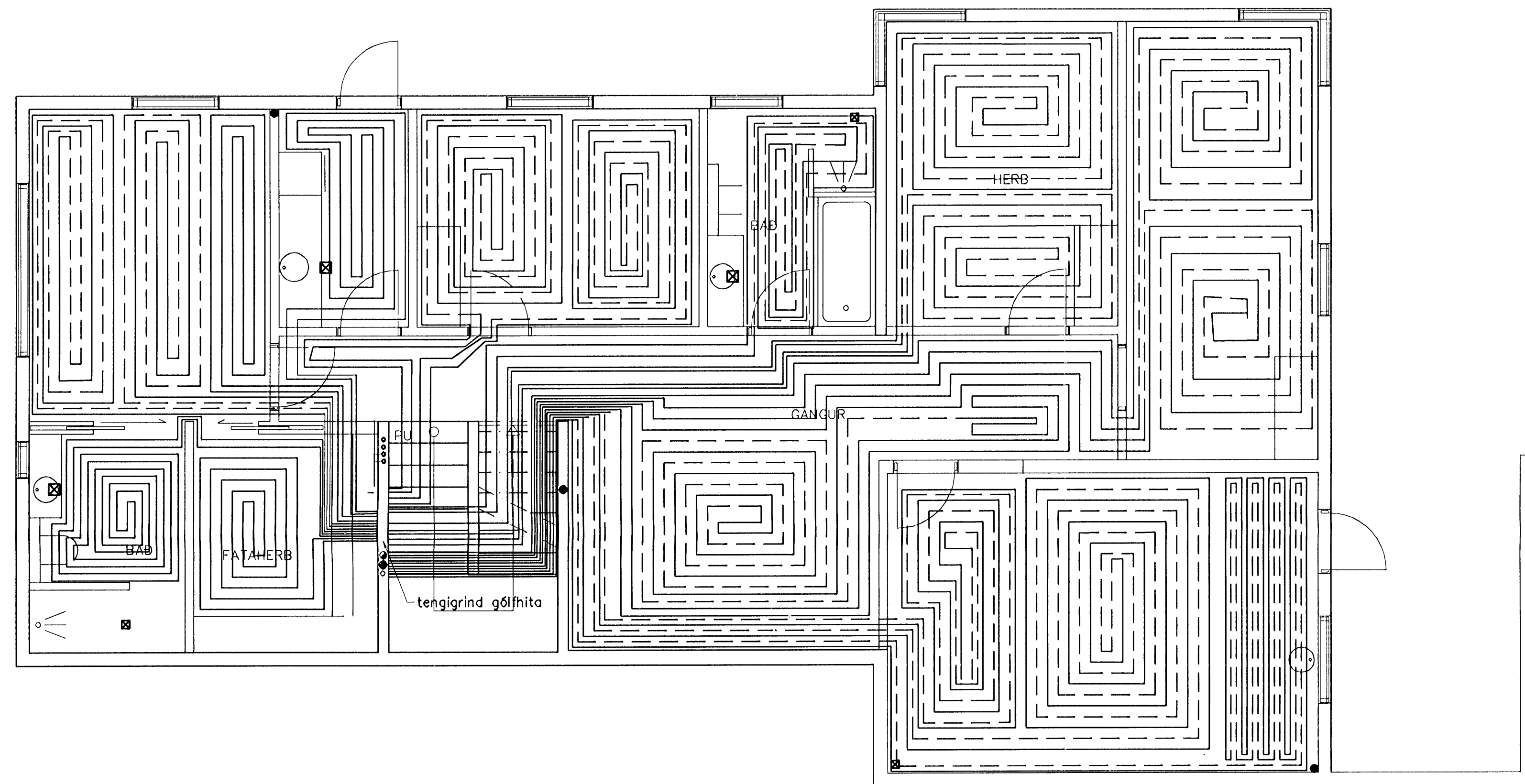
GRUNNMYND 1 HÆÐAR 1:50
