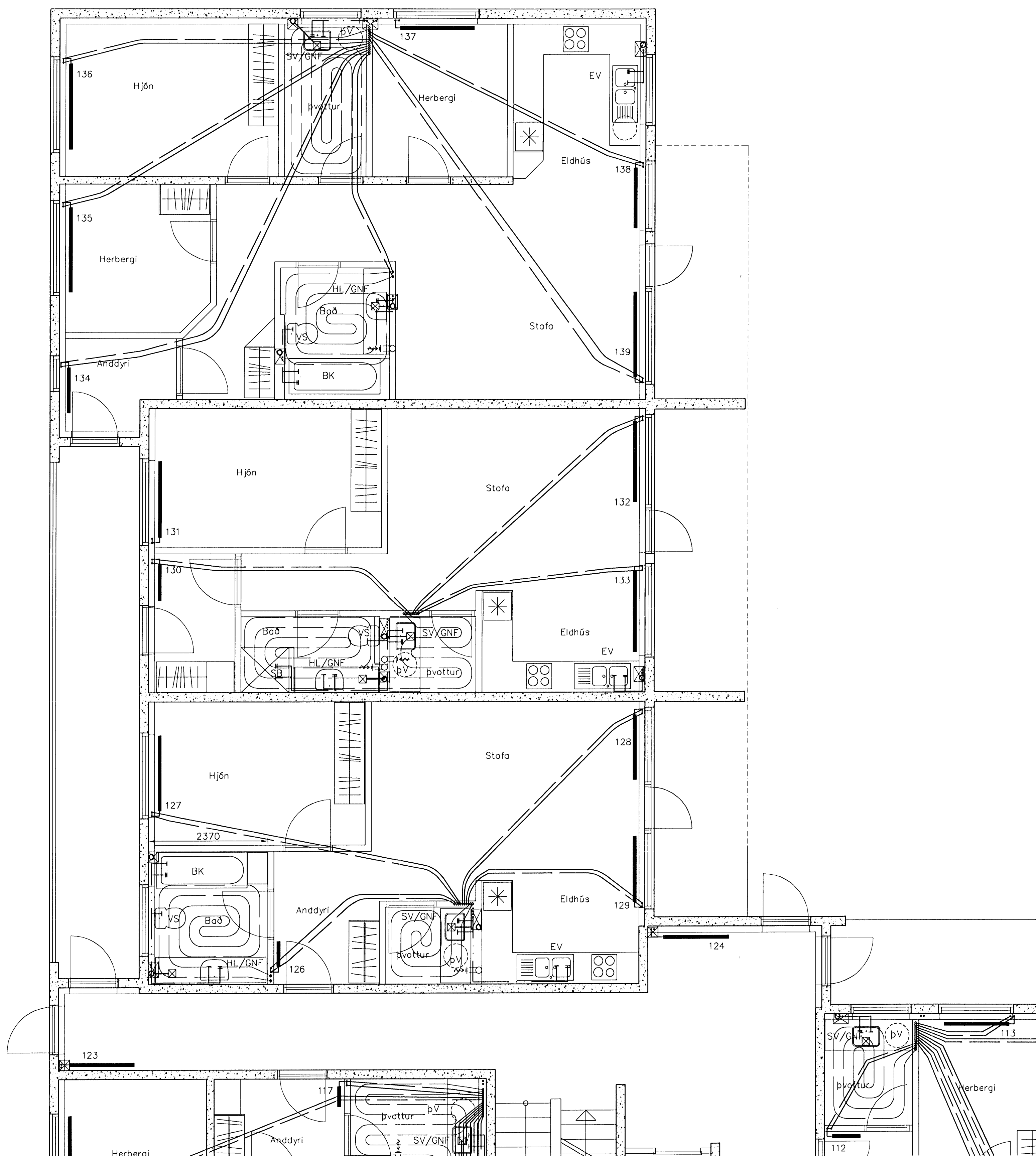
Lagnir 1. hæð, 1:50
