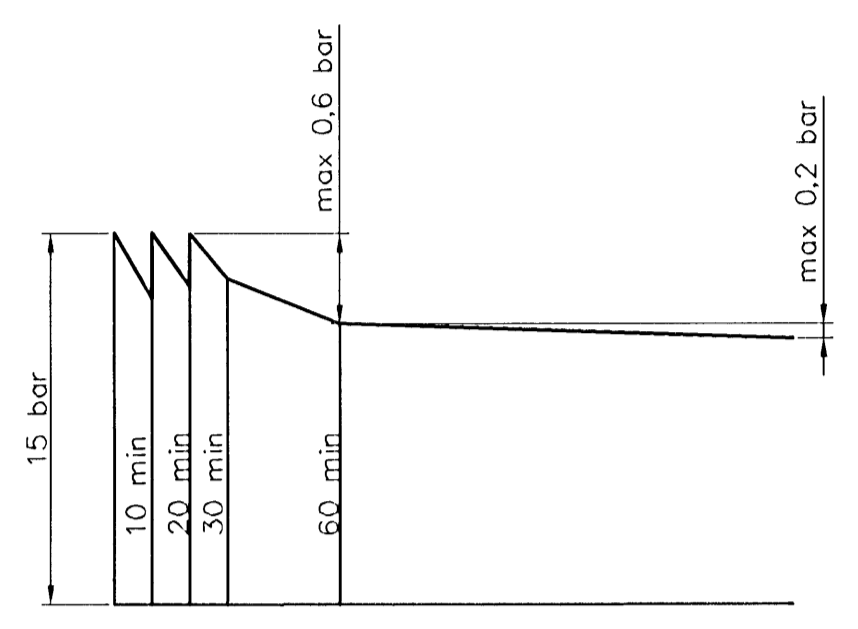
Þrjústípröfun á neysluvatnslögnum línurit
