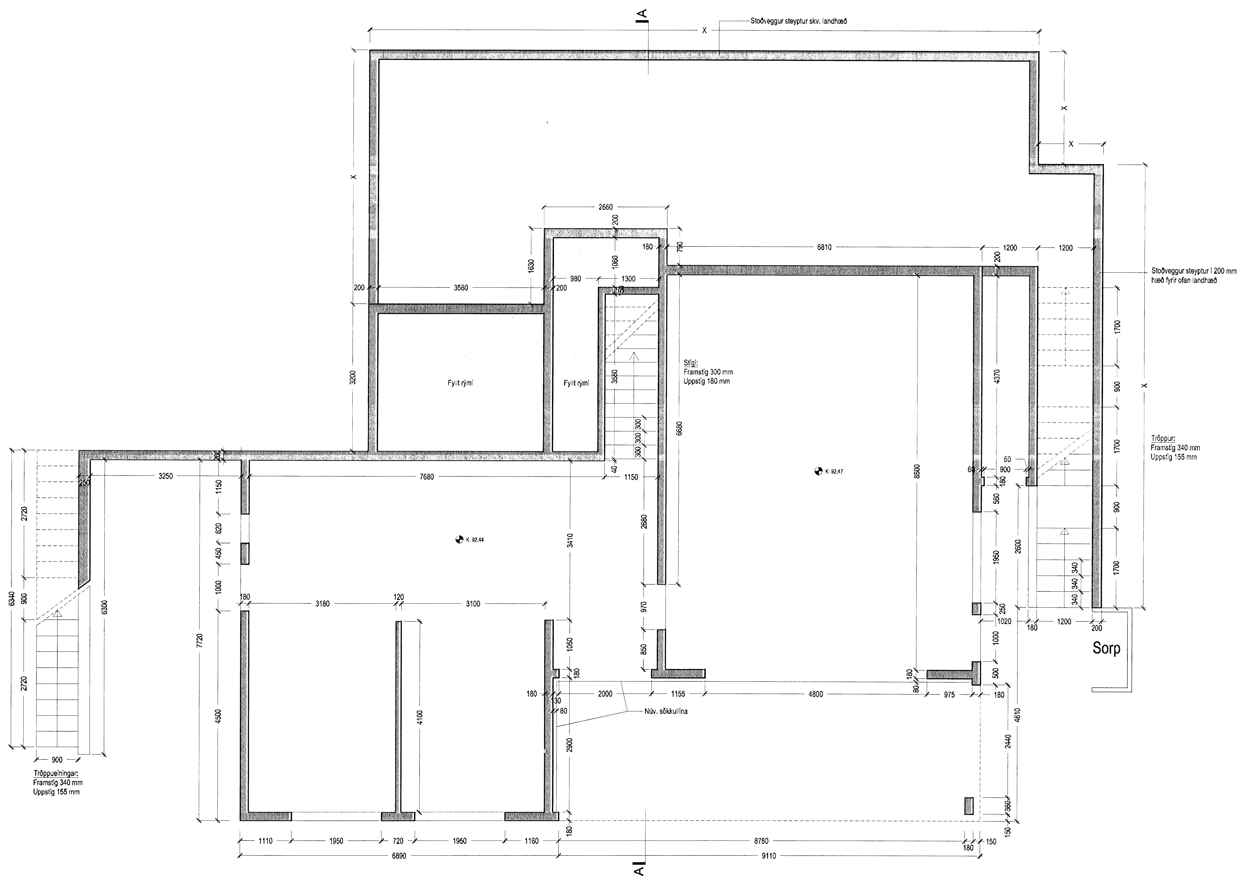
GRUNNMÝND 1. HÆÐAR í mkv. 1:50
