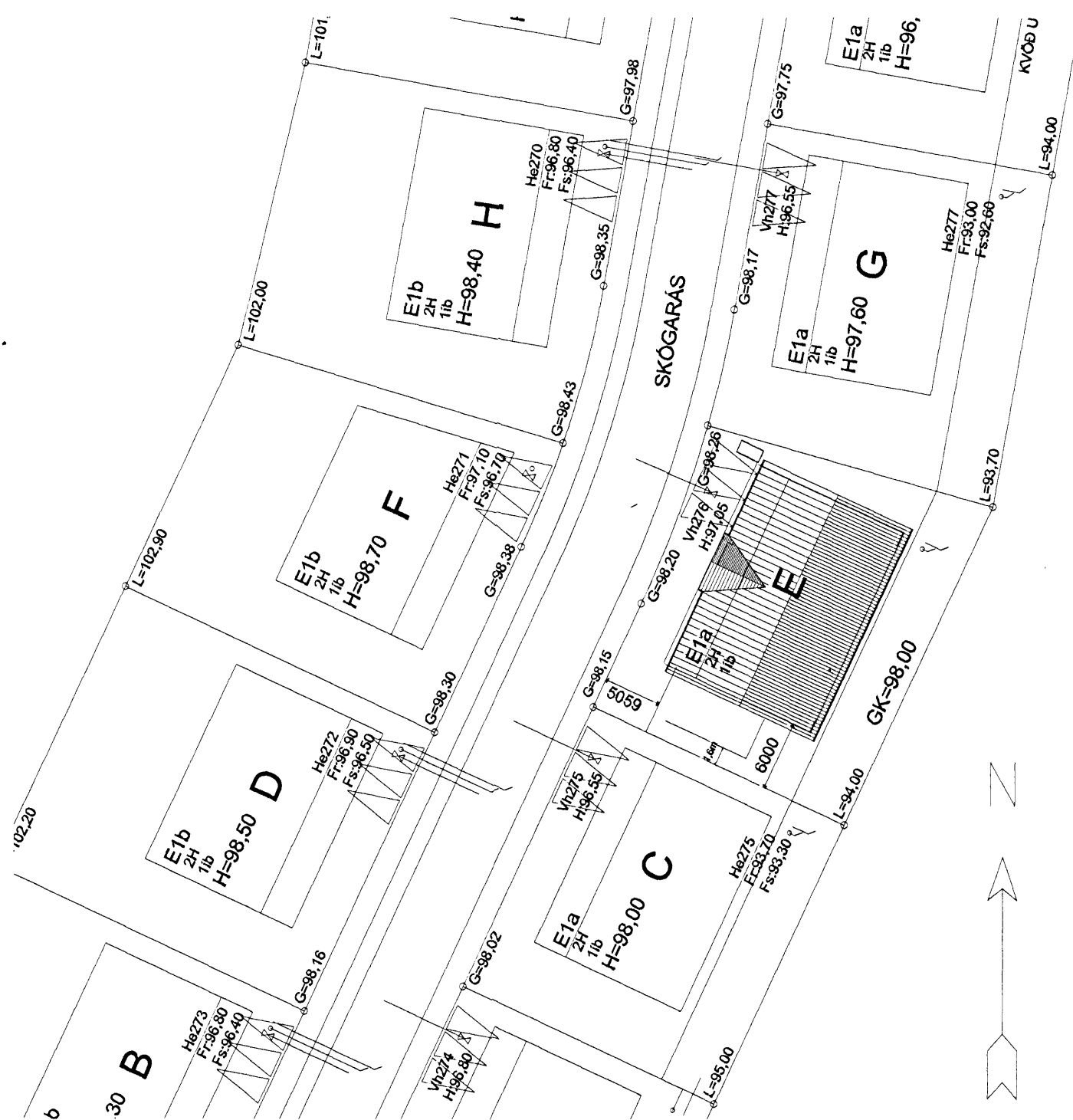
AFSTÖÐUMYND 1:500
