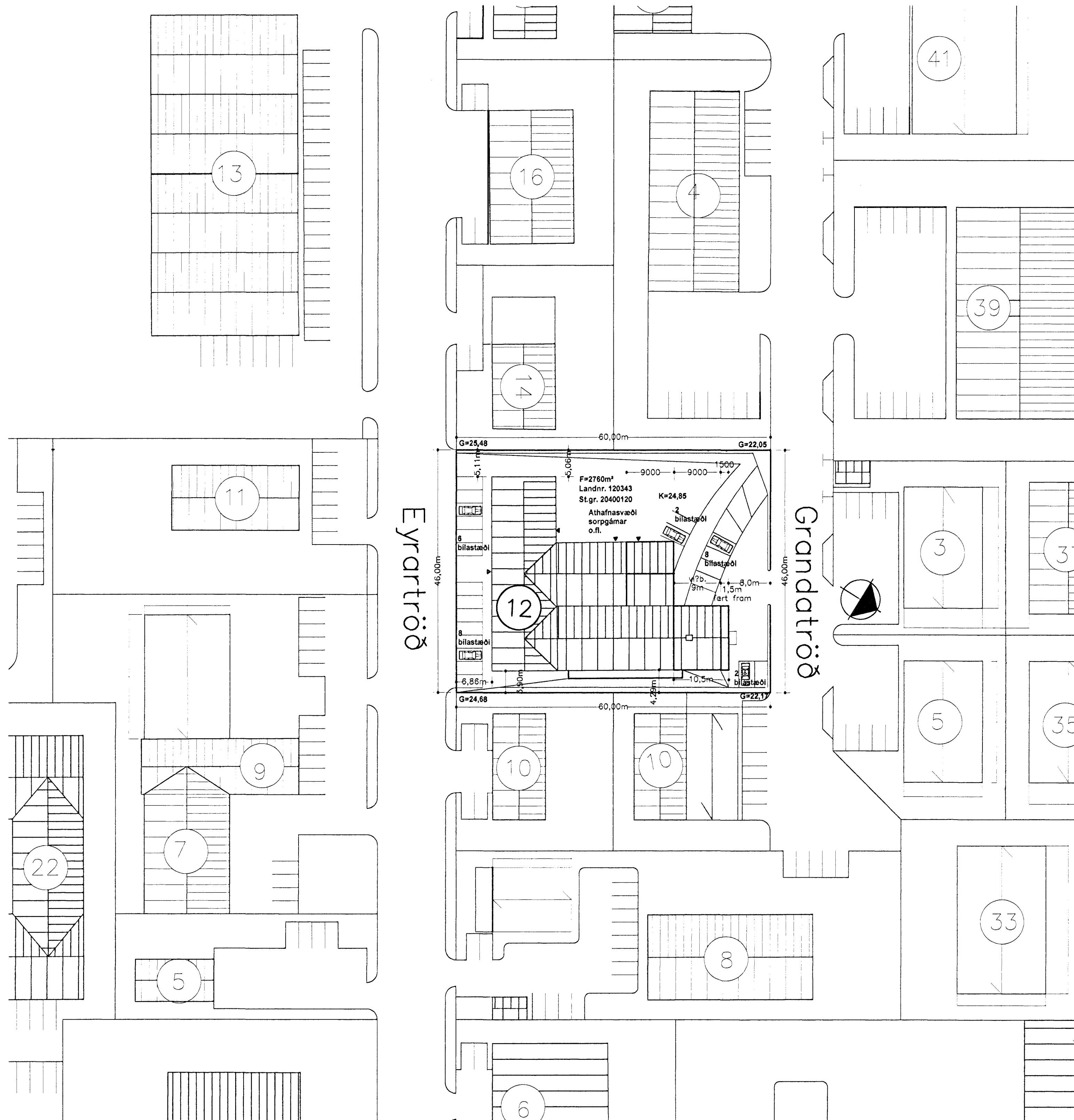
Afstöðumynd mkv. 1:500
