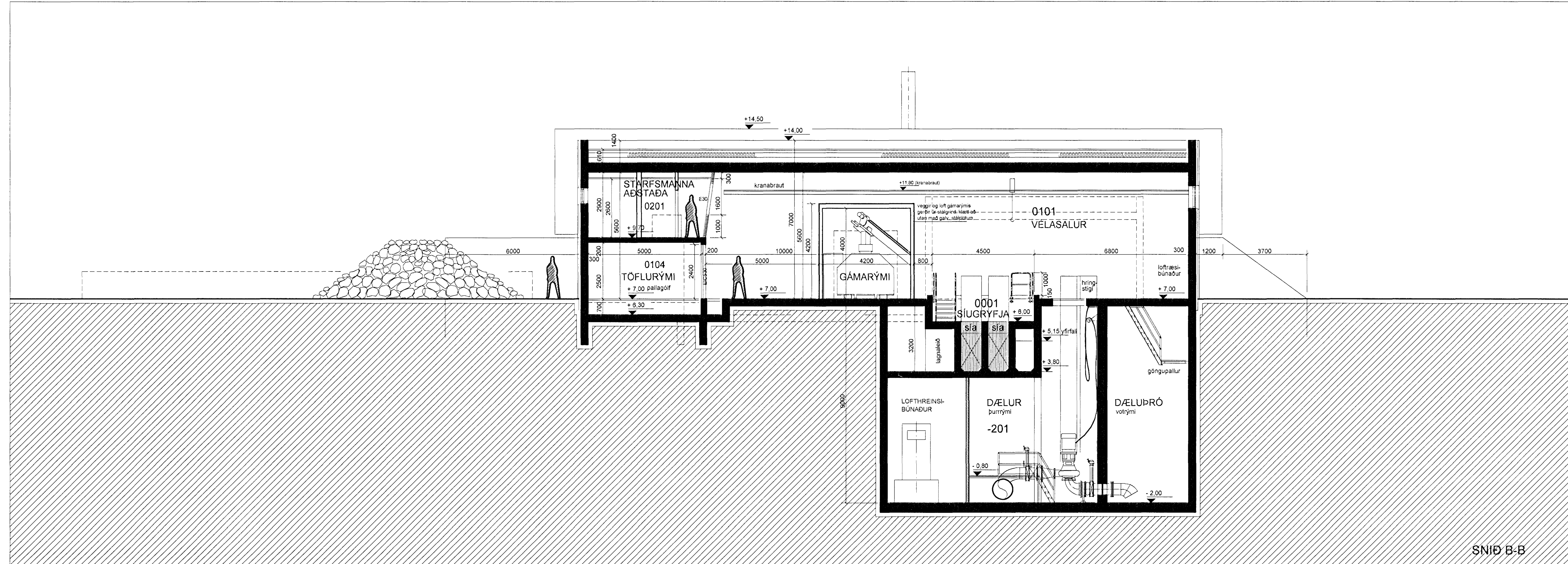
SNÍÐ A-A
