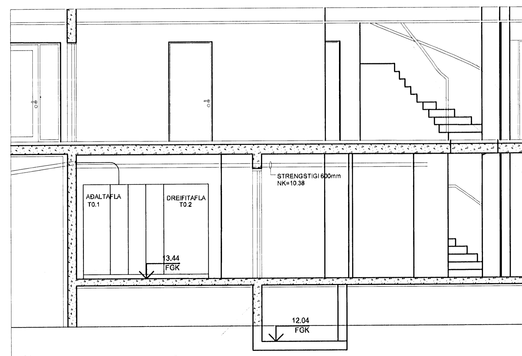
SNÍÐ A-A Í TÖFLUHERBERGI MKV. 1:50
