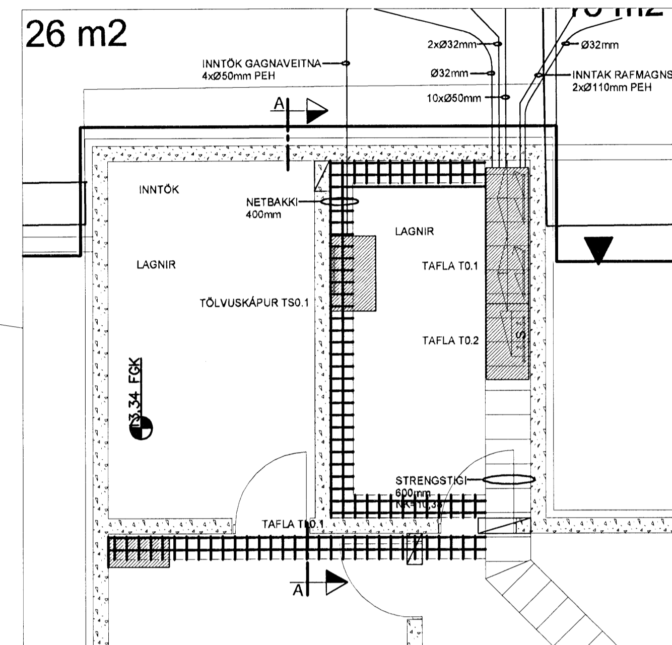
GRUNNMYND AF INNTAKI OG ADALTÖFLUHERB. MKV. 1:50
