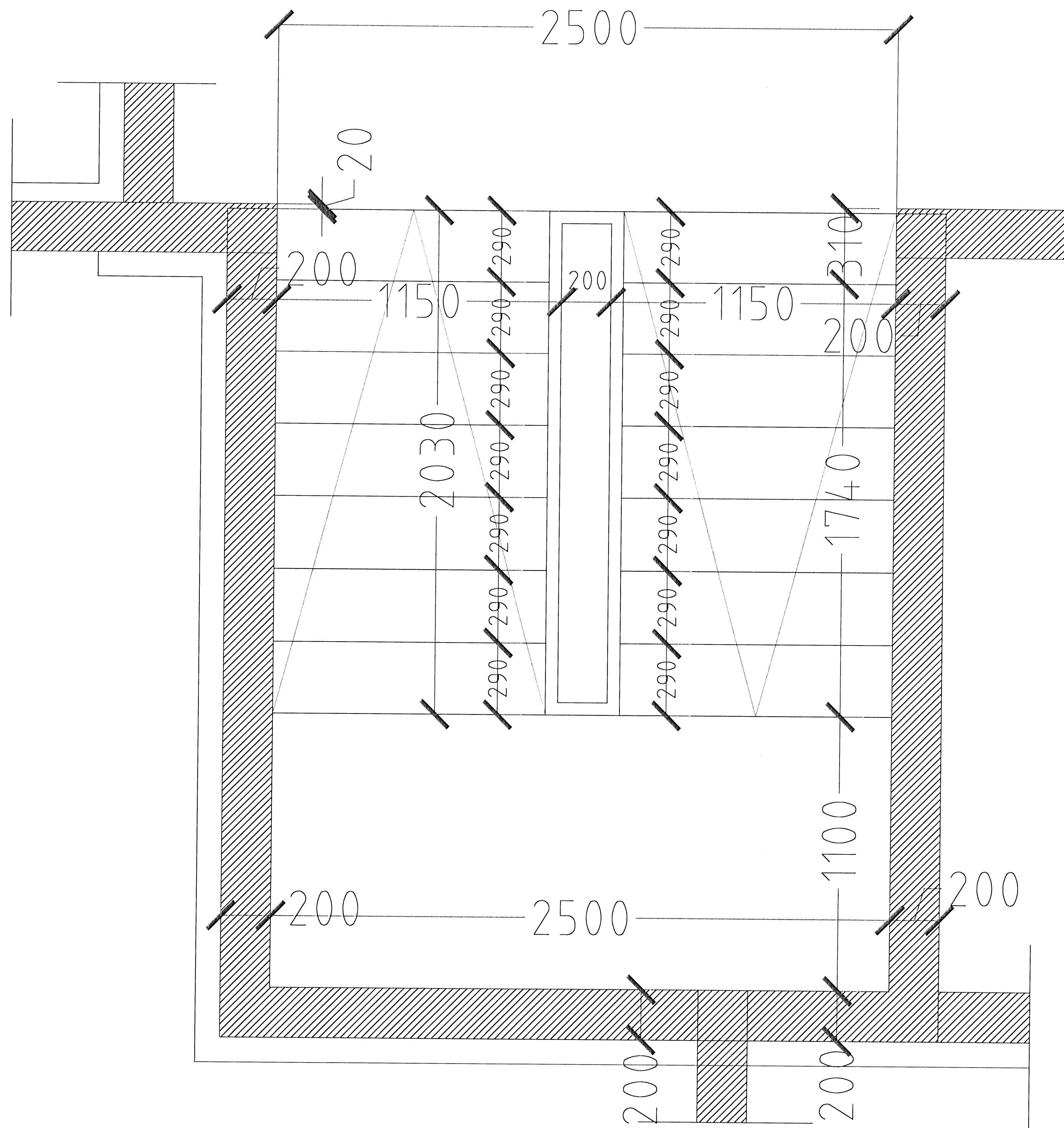
GRUNNMYND STIGI MKV. 1:10. 1. 2 og 3 HÆÐ.
