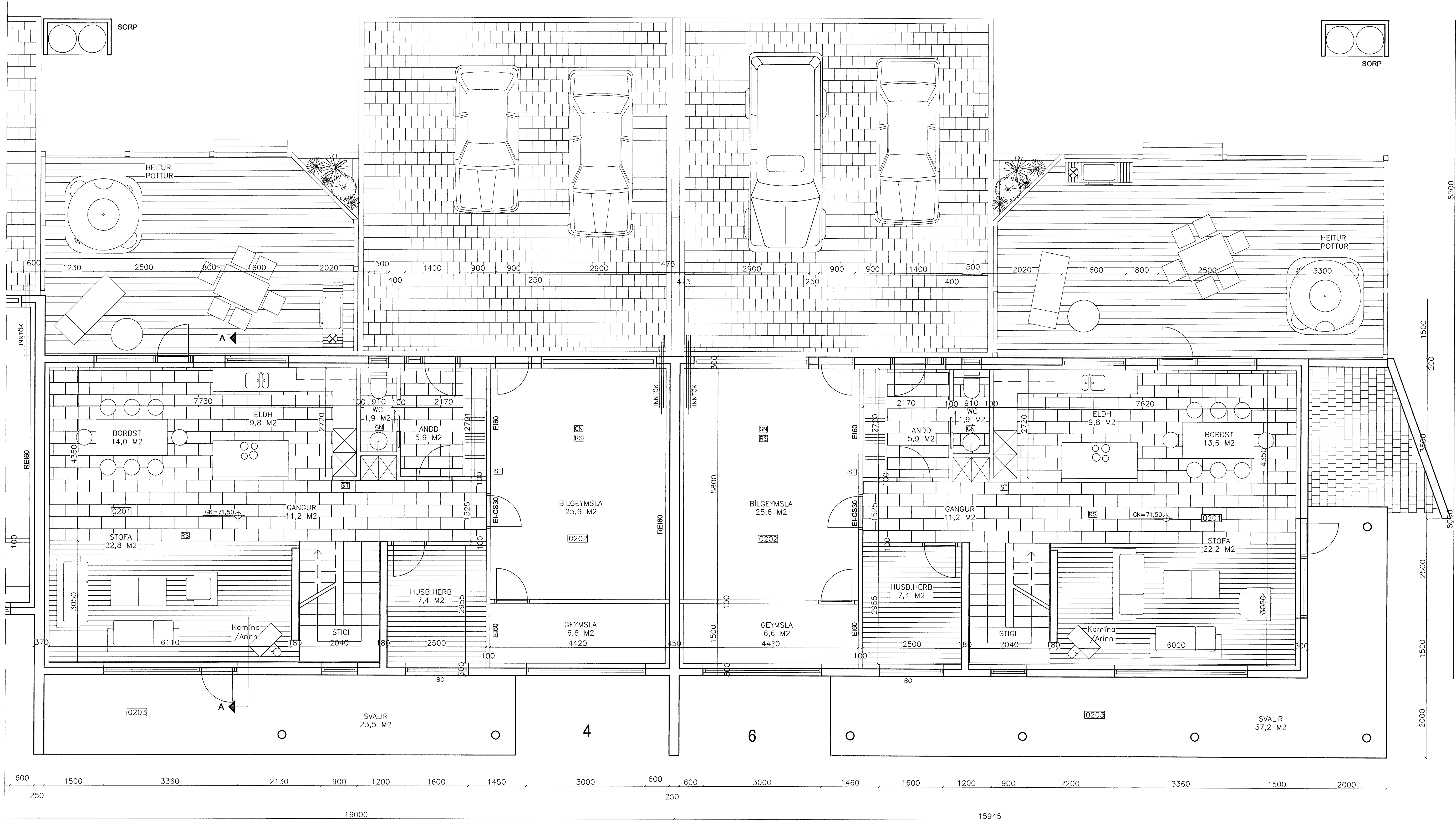
GRUNNMYND 2. hæð
