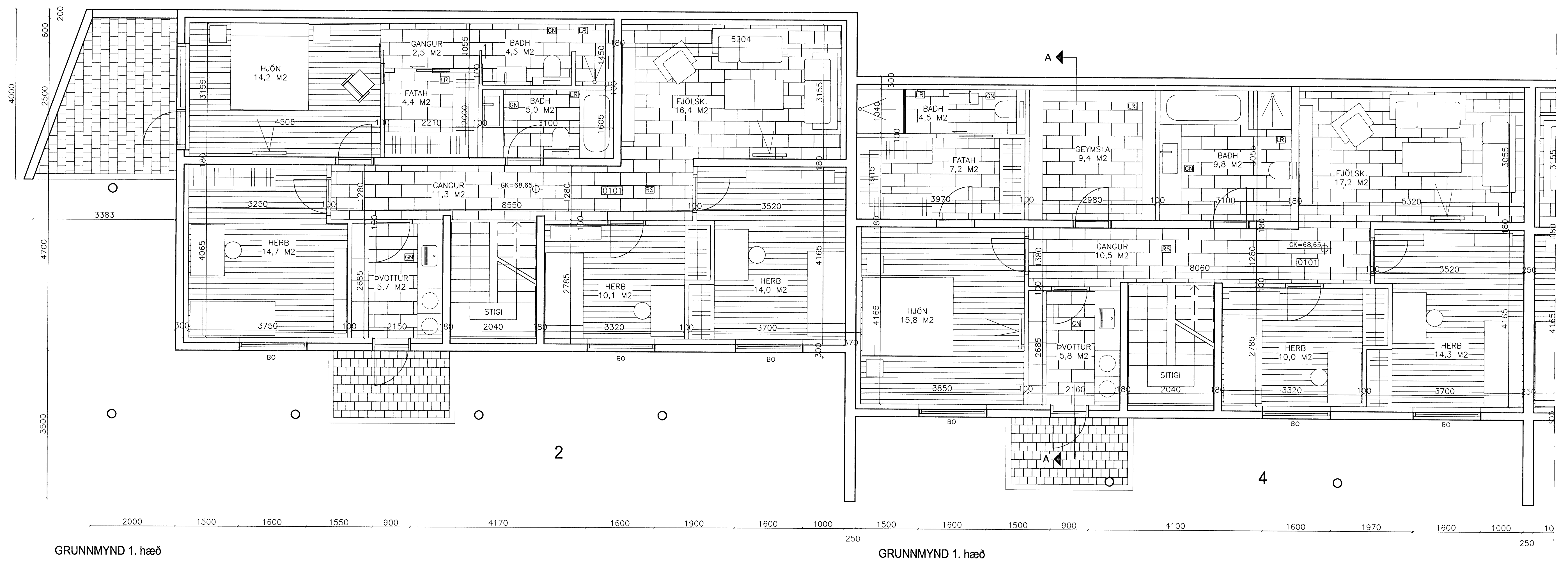
GRUNNMYND 1. hæð
