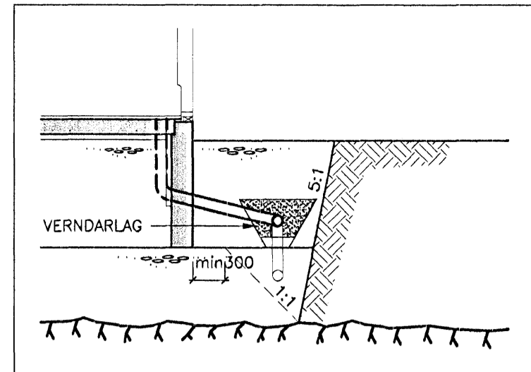
SNID VÍÐ SÖKKUL Mkv. 1:50
